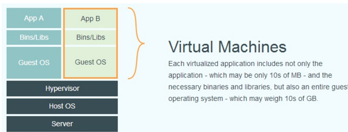
图 1.4.1.1 - 传统虚拟化
