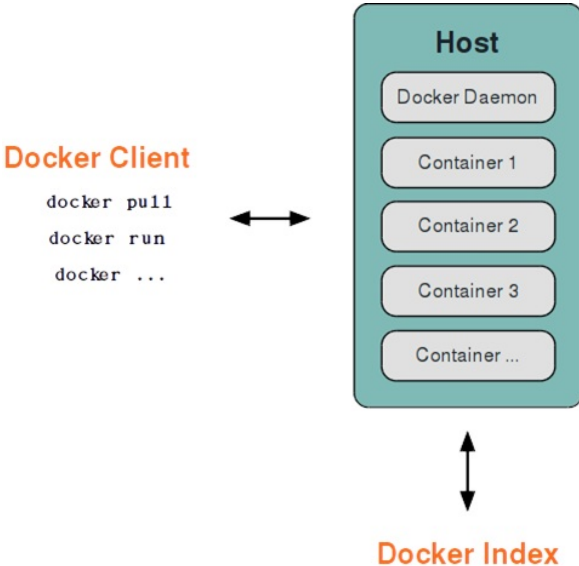
图 1.18.1.1 - Docker 基本架构
