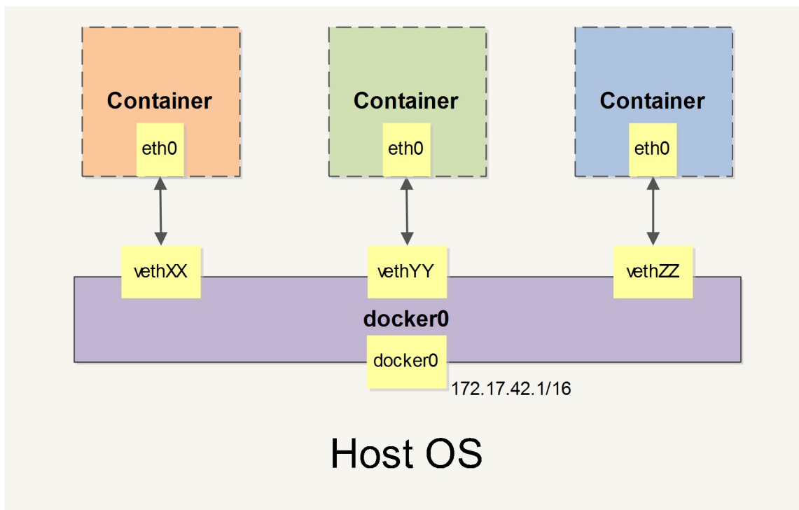
图 1.12.1 - Docker 网络
