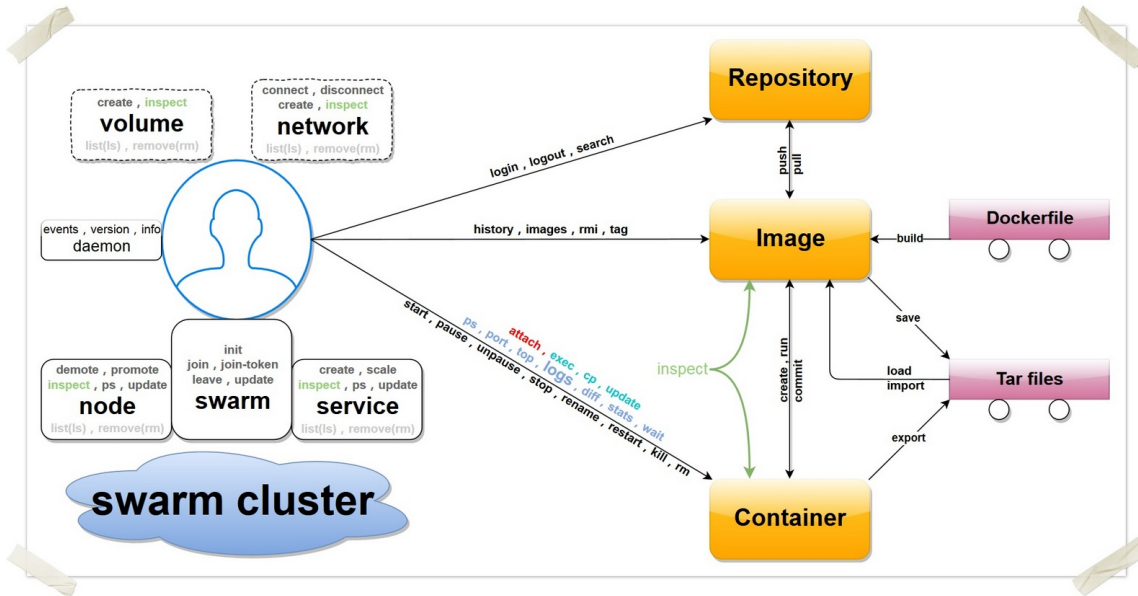
图 1.27.3.1 - Docker 命令总结
