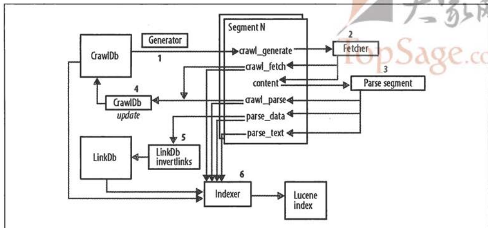
图 16-5. 分割
