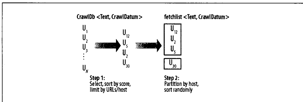
图 16-7. 产生 fetchlist
