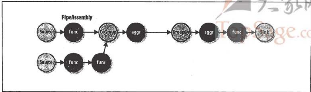
图 16-16. 操作流程
