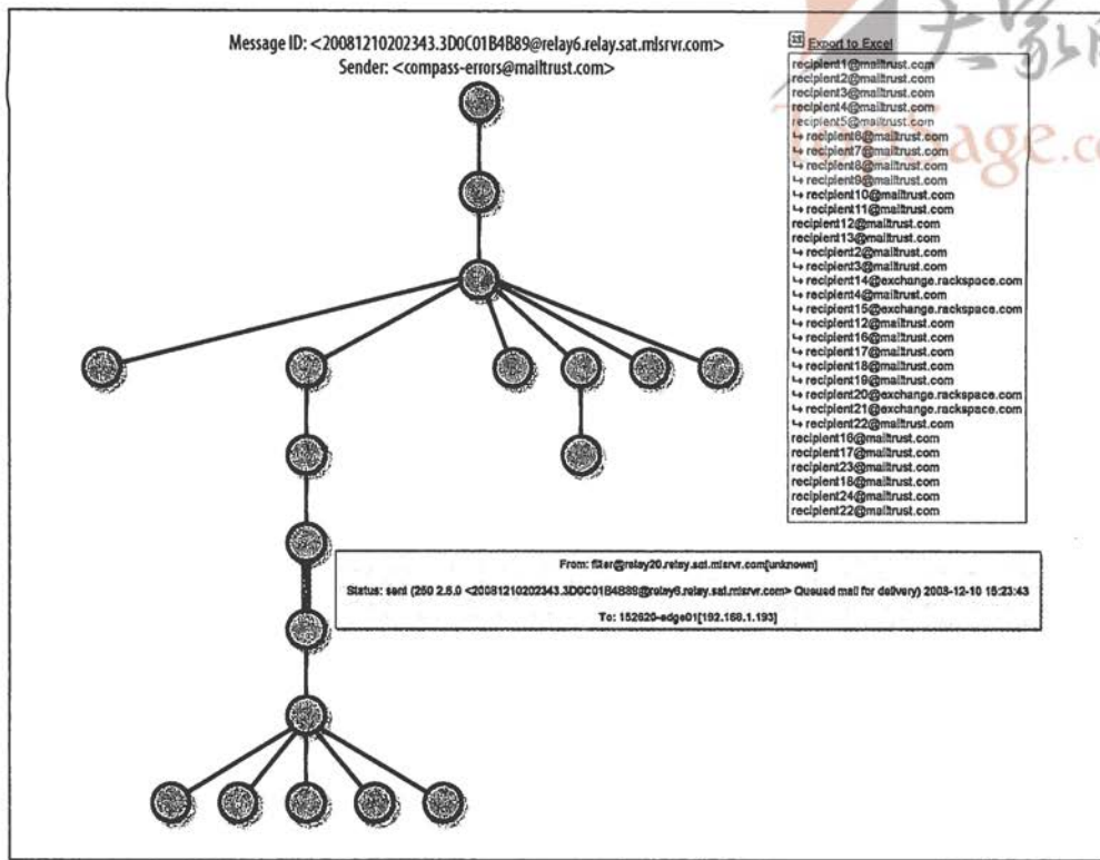
图 16-10. 数据树
