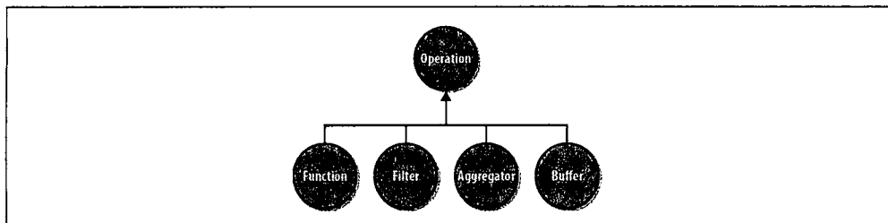
图 16-15. 操作类型
