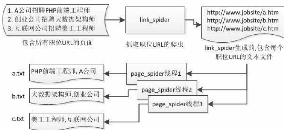
图4.3 两个爬虫的工作过程
