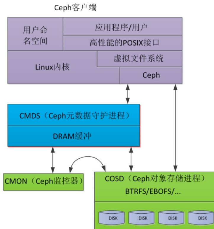
图9.10 Ceph内部结构示意图
