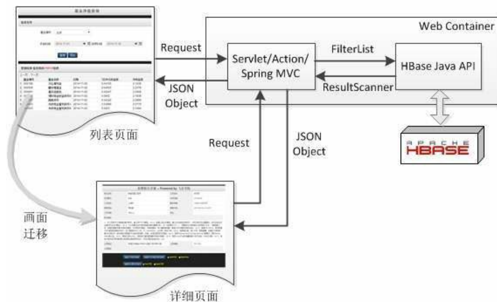
图6.9 前端页面和HBase数据交互过程
