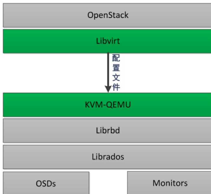
图9.12 OpenStack与Ceph内部连接关系图
