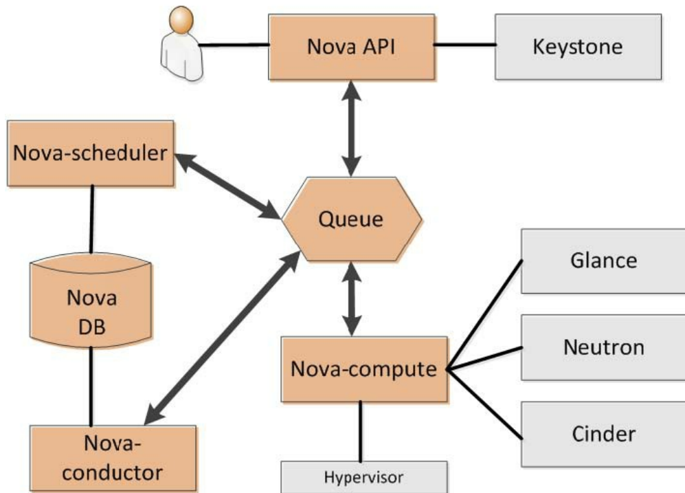
图9.5 Image组件工作原理示意图
