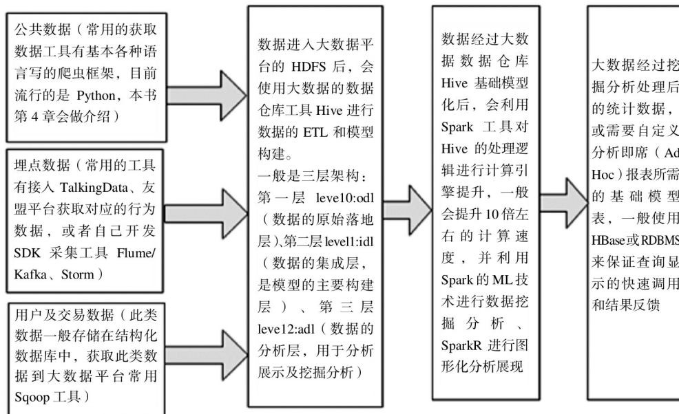
图3.1 大数据系统的数据流图及组件
