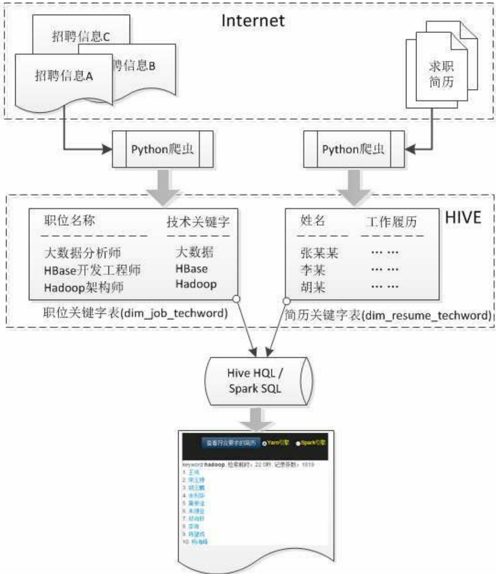
图8.2 自动匹配简历过程示意图
