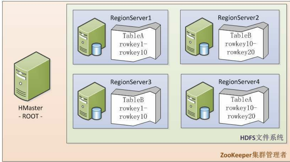
图6.1 HBase数据存储示意图
