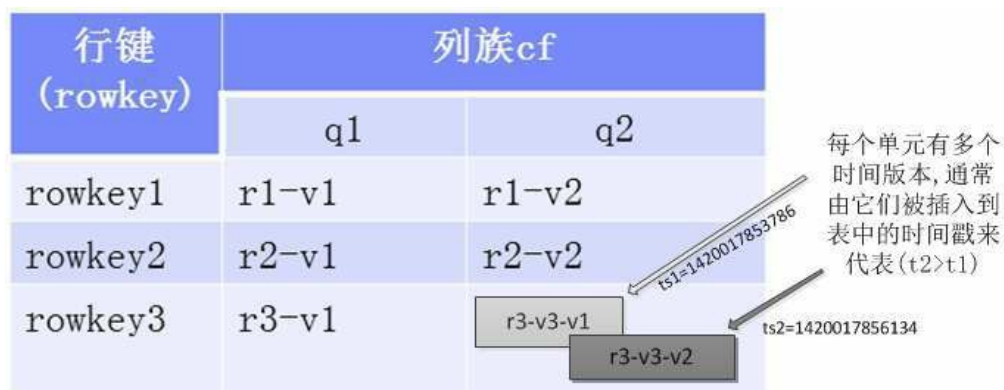
图6.3 保存两个不同版本的数据示例
