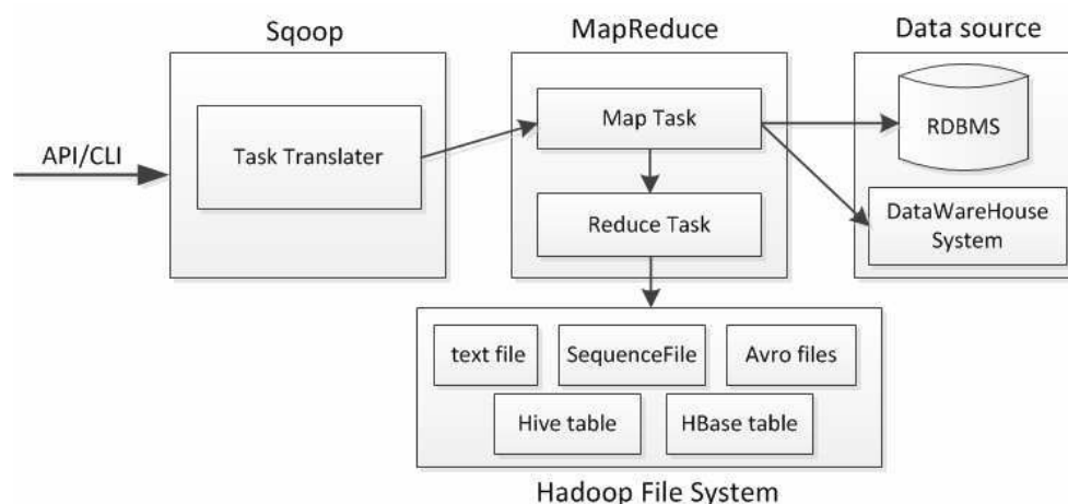
图4.4 Sqoop数据处理流程图
