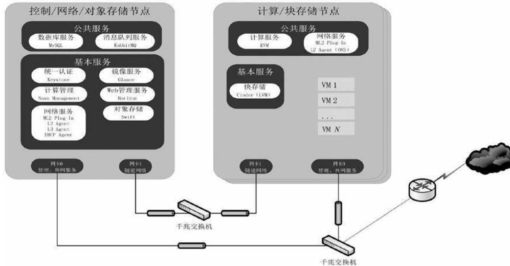
图9.1 一期云基础平台架构图
