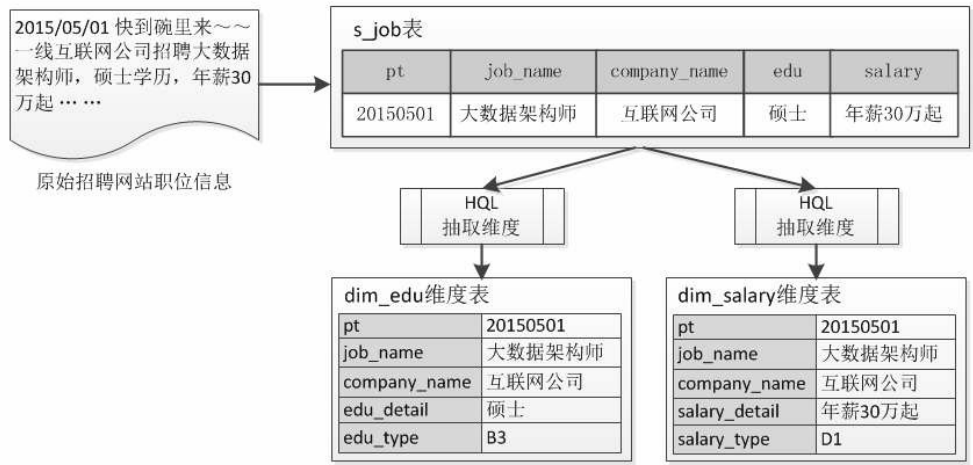
图5.6 从s_job表到维度表的数据流向图
