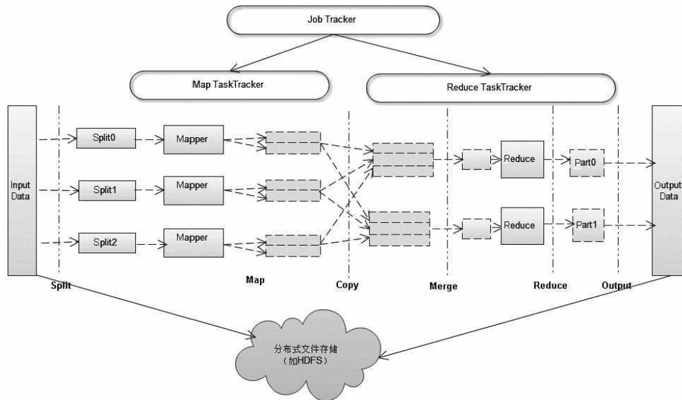
图2.4 MapReduce数据处理架构图
