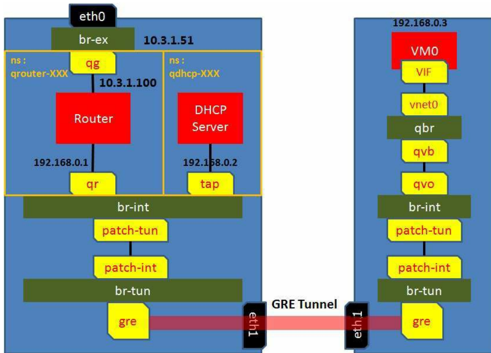
图9.9 采用GRE模式的网络数据交互流图
