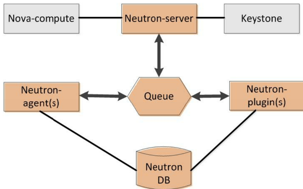
图9.8 Networking工作原理示意图
