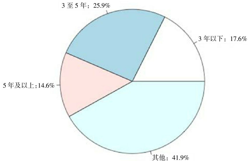
图7.3 统计图形
