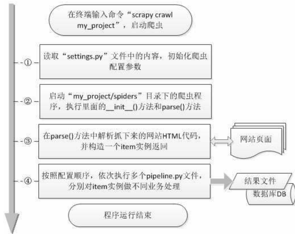
图4.2 Scrapy爬虫的执行过程
