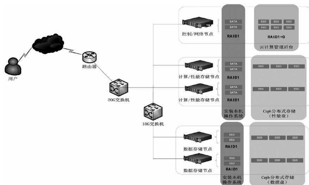
图9.3 服务器资源规划图
