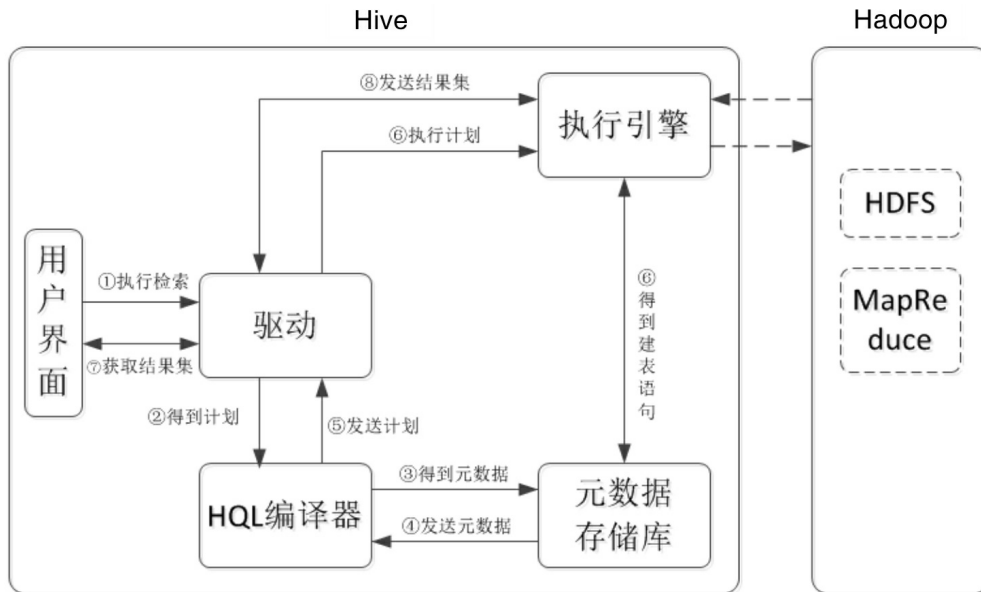
图5.1 Hive和Hadoop之间的内部依赖关系（图片摘自 https://cwiki.apache.org/confluence/display/Hive/Design ，并有所简化）
