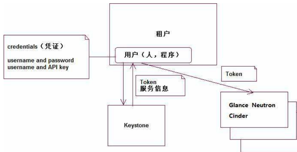
图9.4 Identity组建工作原理示意图
