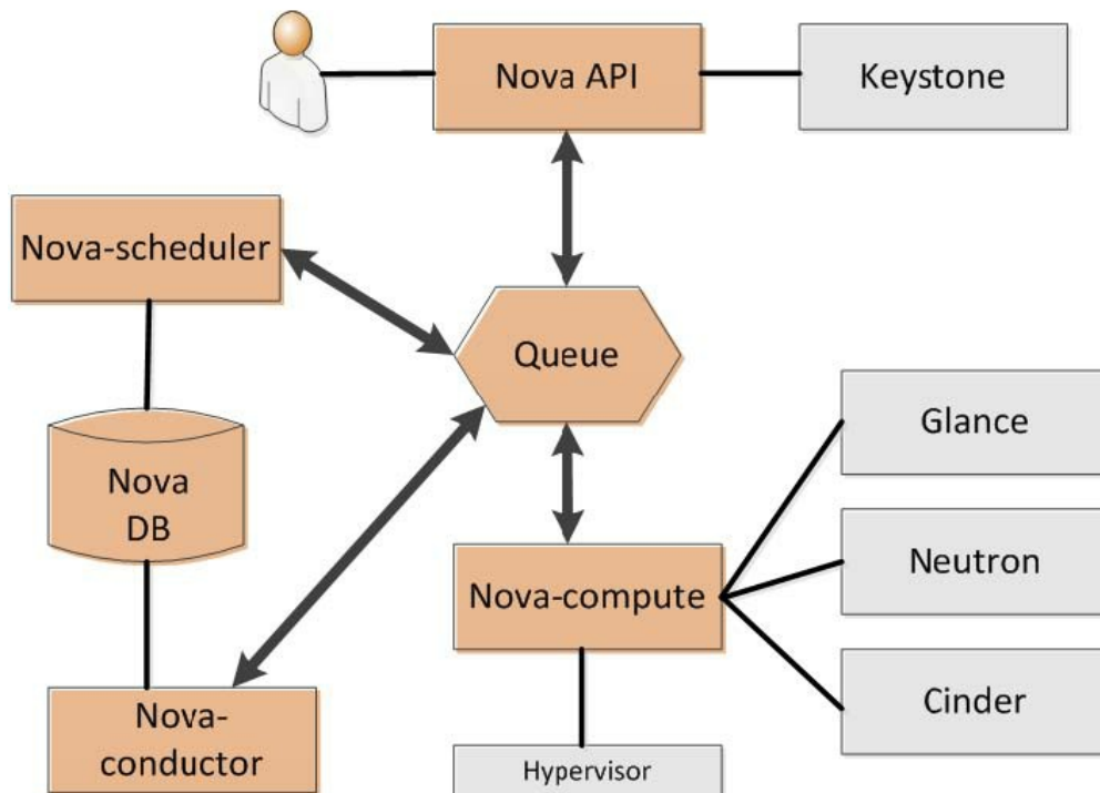
图9.6 Compute组件工作原理示意图
