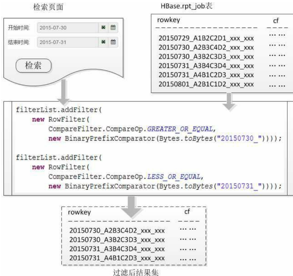
图6.7 按照职位发布时间筛选数据的处理过程
