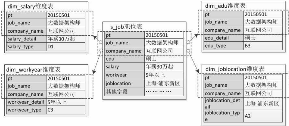
图5.8 s_job表左外连接的过程
