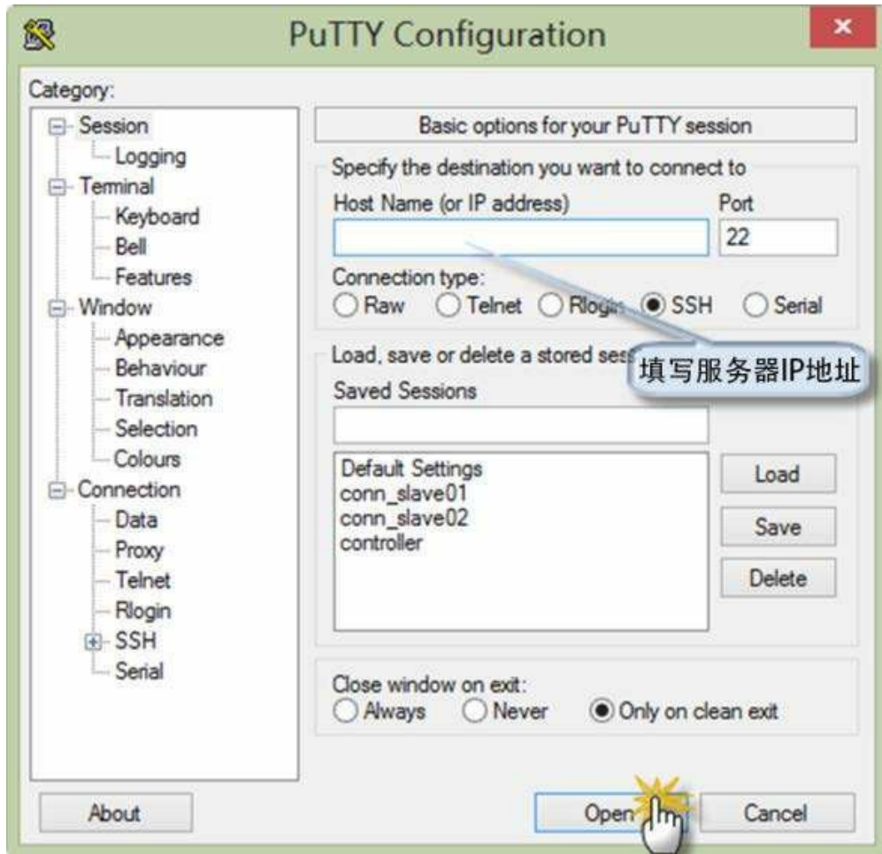
图2.2 PuTTY配置
