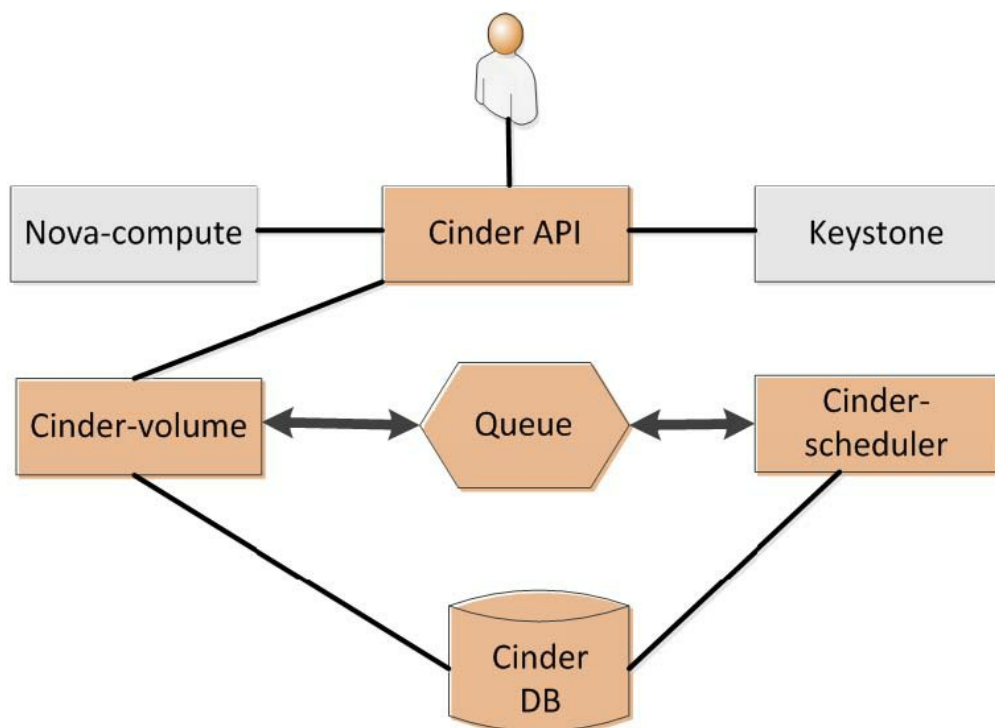
图9.7 Storage组件工作原理示意图
