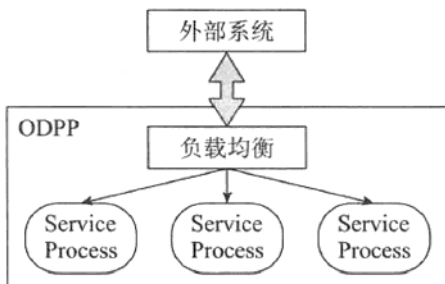
图8-4 ODDP访问接入结构
