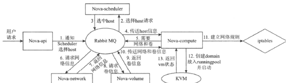
图16-9 Nova在各组件之间的消息传递流程
