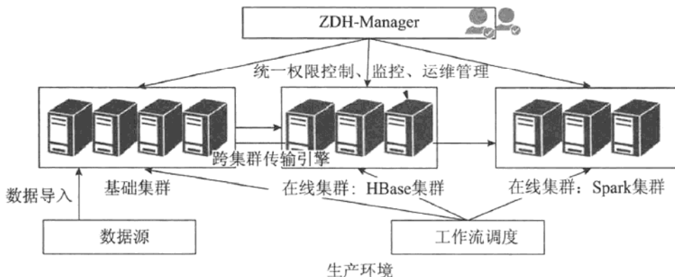
图12-4 混合型组网模式图
