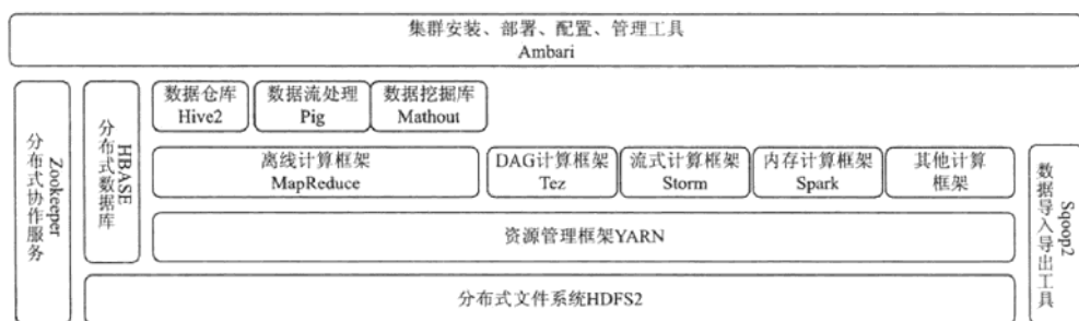
图4-2 Hadoop2.0生态系统图
