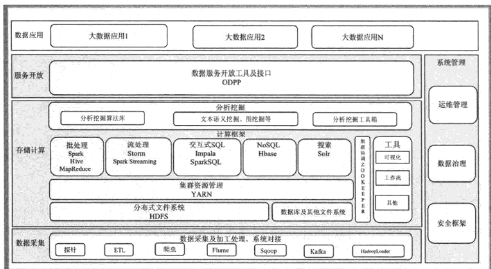
图13-1 DAP总体架构图
