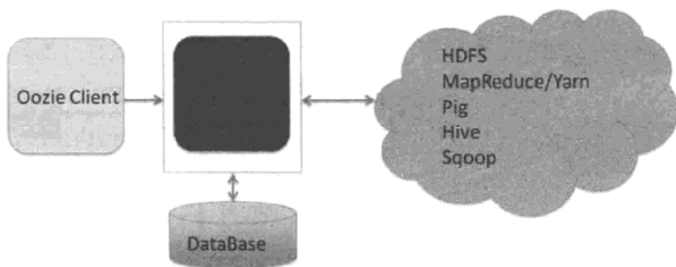
图5-10 Oozie架构图
