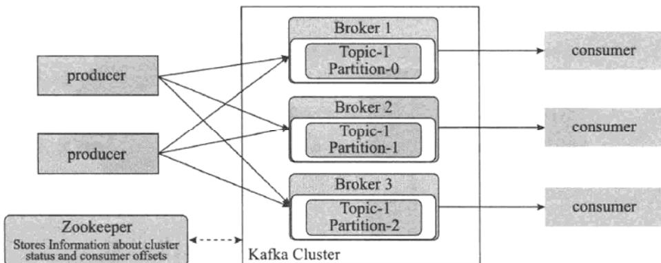
图5-11 Kafka架构图
