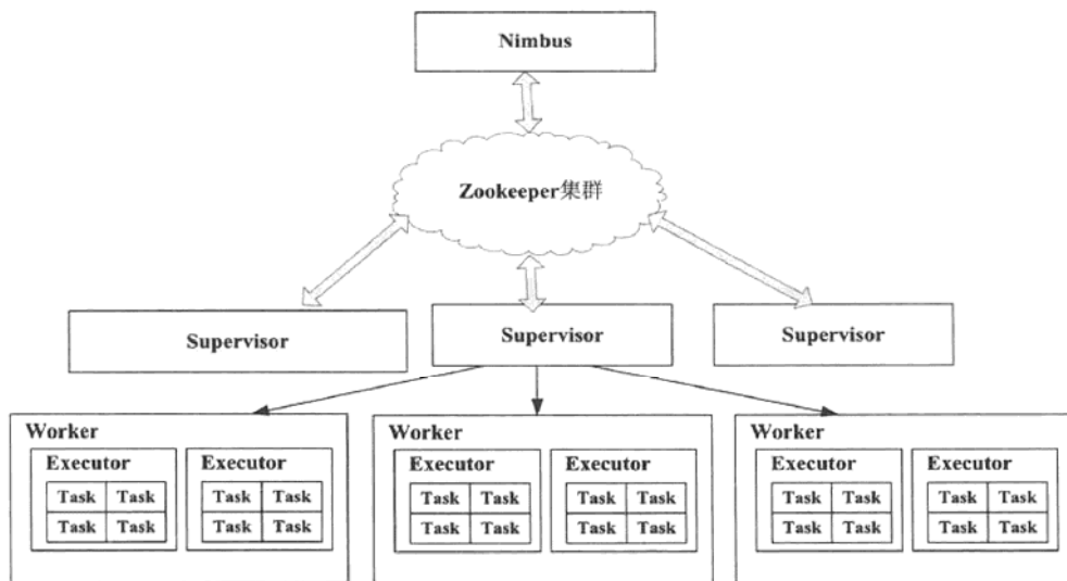
图5-5 Storm架构图
