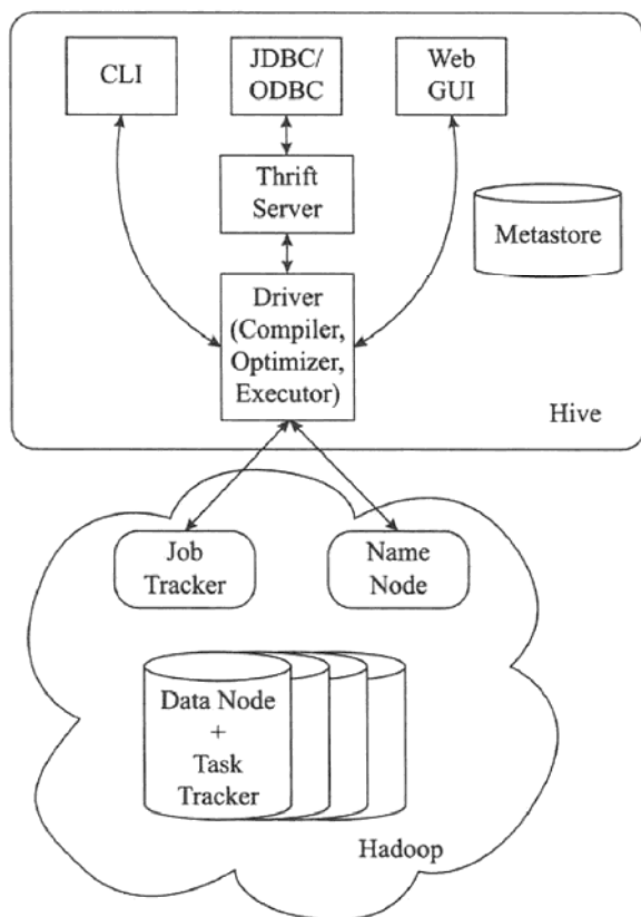
图5-1 Hive架构图
