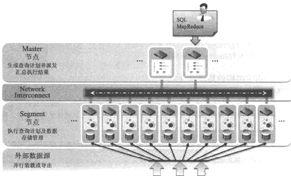
图15-5 Greenplum架构图
