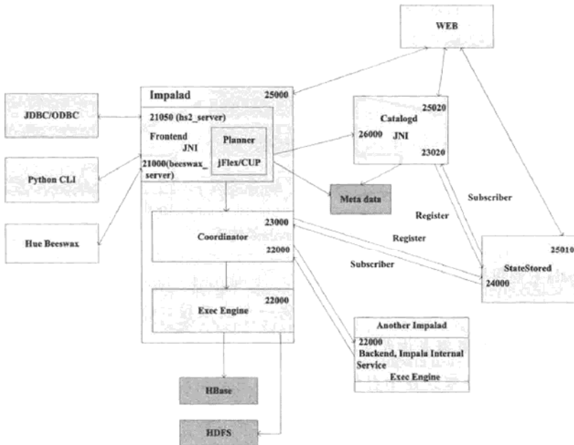
图5-9 Impala内部流程图
