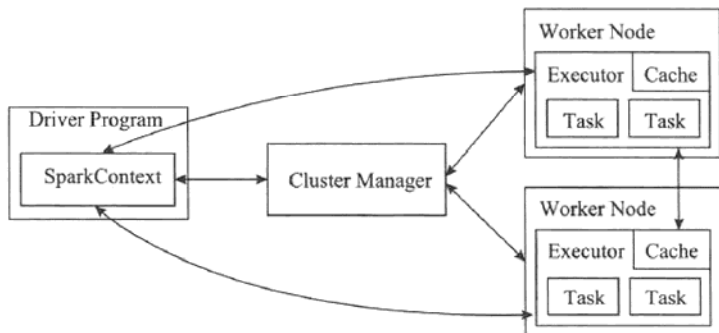
图6-3 Apache Spark在集群环境中的运行框架
