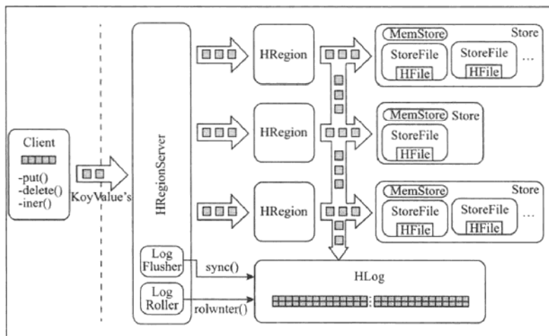
图5-4 HBase物理存储示意图
