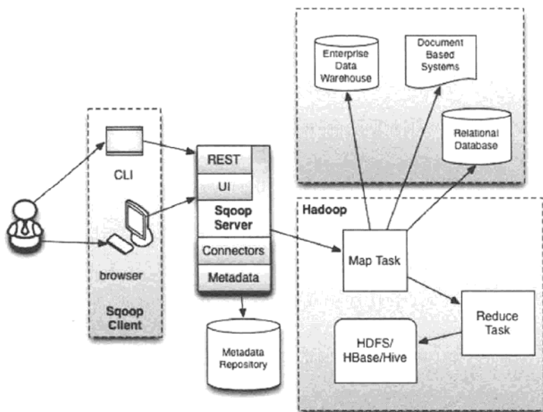
图5-12 Sqoop2架构图
