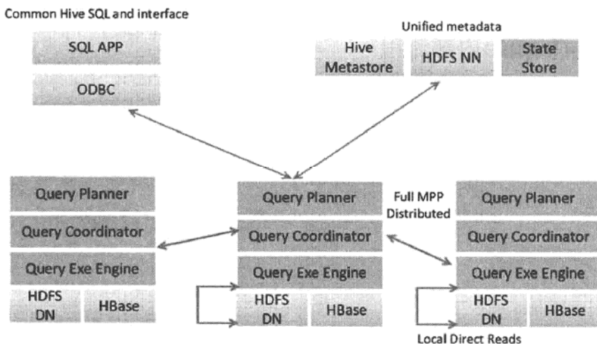
图5-8 Impala架构图
