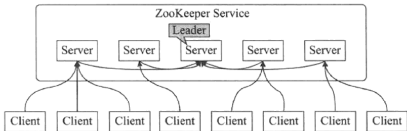
图4-9 ZooKeeper架构图
