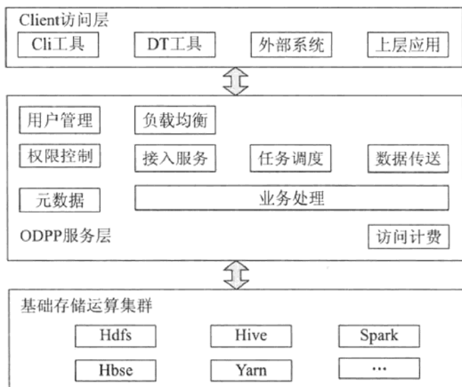
图8-2 ODPP架构图
