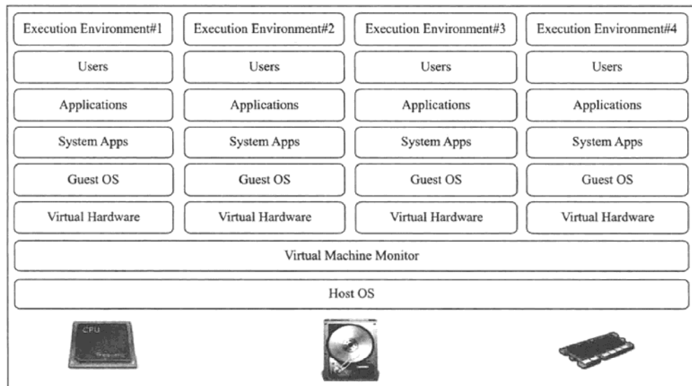
图16-3 虚拟机部署
