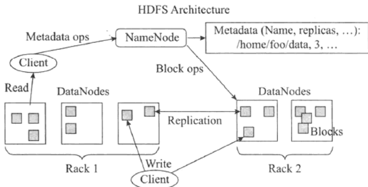
图4-3 HDFS架构图
