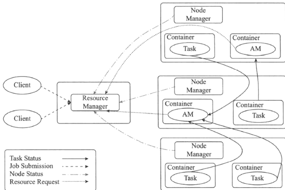
图4-5 YARN架构图
