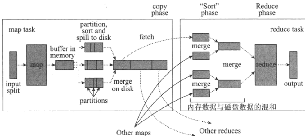
图4-8 MapReduce处理流程图
