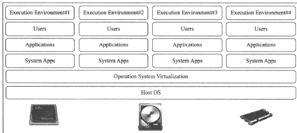
图16-5 虚拟专用服务器部署
