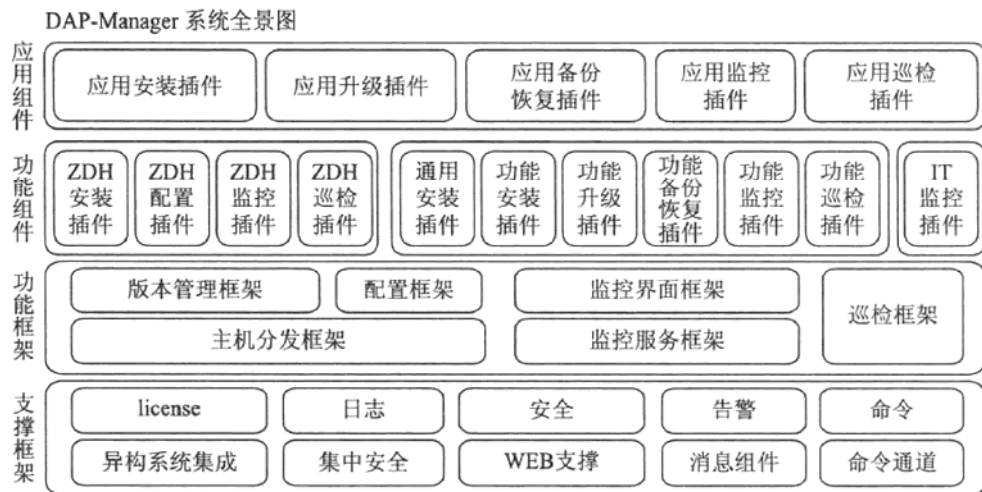
图11-6 DAP-Manager 软件框架图
