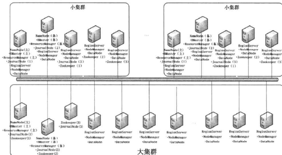
图13-5 某集团的实际部署图
