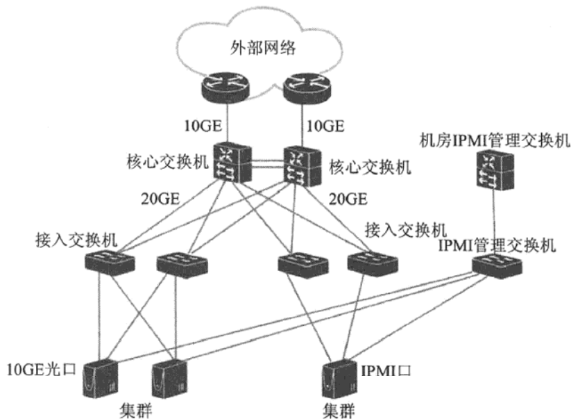
图12-3 双网双平面的网络部署模式
