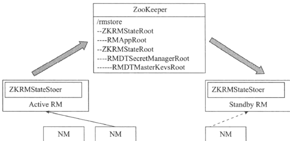
图4-11 ZooKeeper在YARN中的应用示意图
