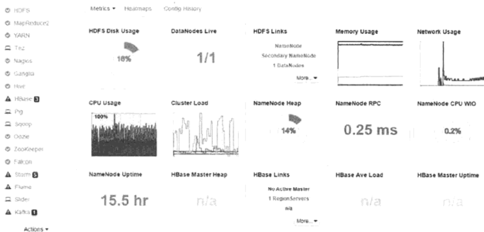
图11-3 Ambari的用户界面效果图
