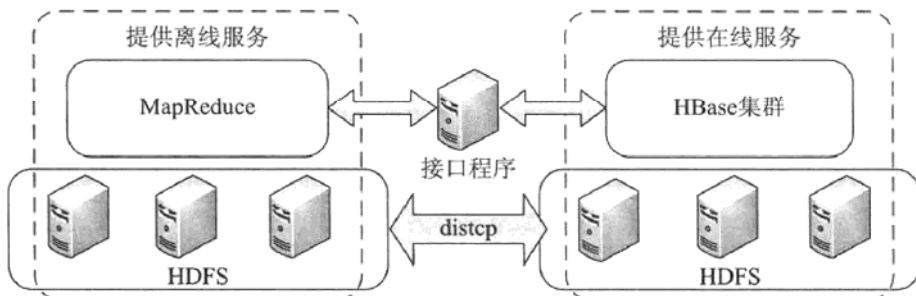
图13-3 资源隔离集群的数据迁移方式
