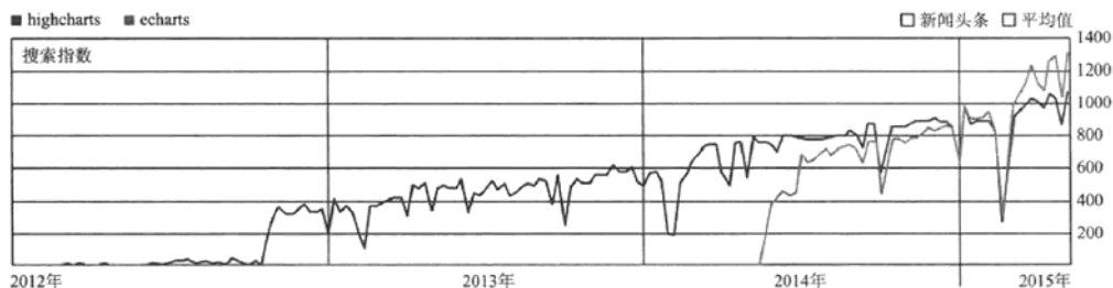
图9-5 highcharts和ECharts在百度指数的对比分析
