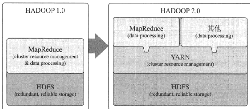
图4-1 Hadoop版本演进图
