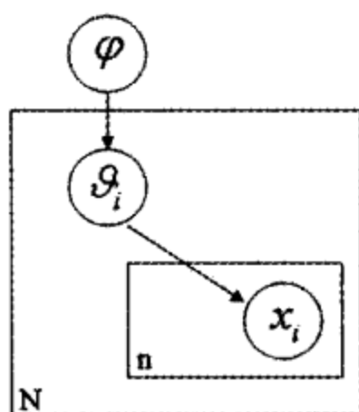
层级贝叶斯
