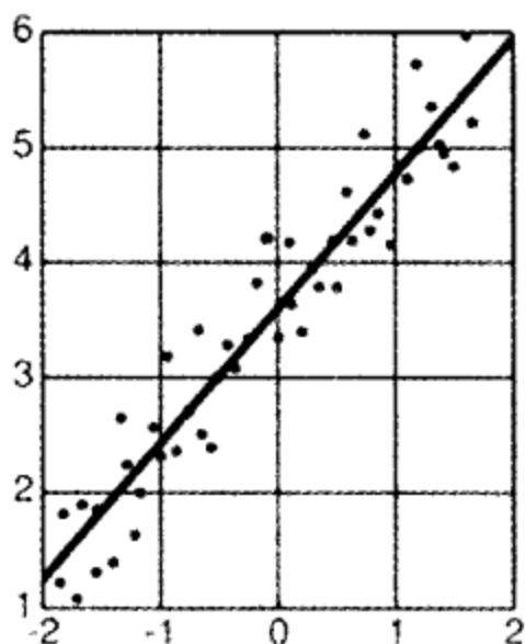
最小二乘
