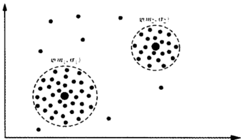
聚类
