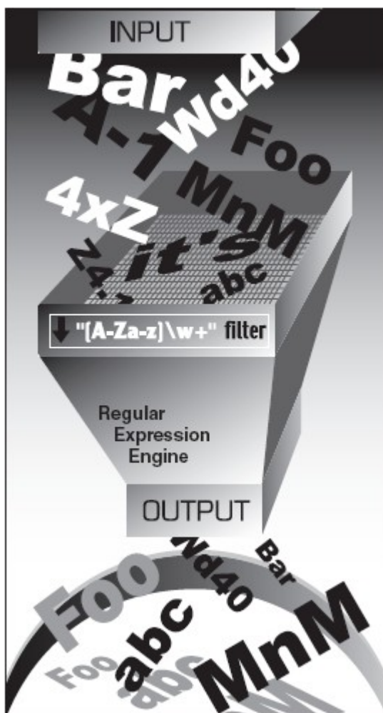
图 15-1 你可以用这个正则表达式匹配有效的 Python 标志符。“ [A-Za-z]\w+ ”的含义是：第一个字符是字母，即，由大写字母 A 到 Z 或是小写字母 a 到 z 组成，它后面至少 (+) 跟有一个由字母或数字组成的字符 ( \w )。如图，你看到有很多字符串被过滤，只有那些符合我们要求的 RE 模式的字符串被筛选出来。比如，“4xZ”，因为它是数字开头的，所以被过滤了。
