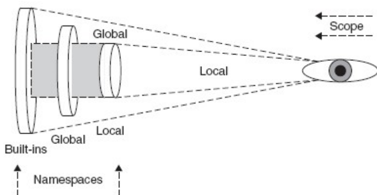
图 12 - 1 名称空间和变量作用域
