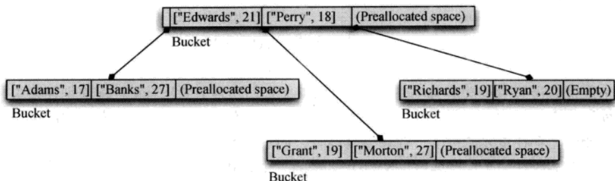
图7-5 B树结构示例
