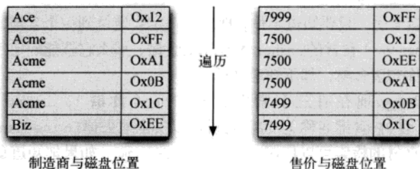
图7-2 单键索引遍历
