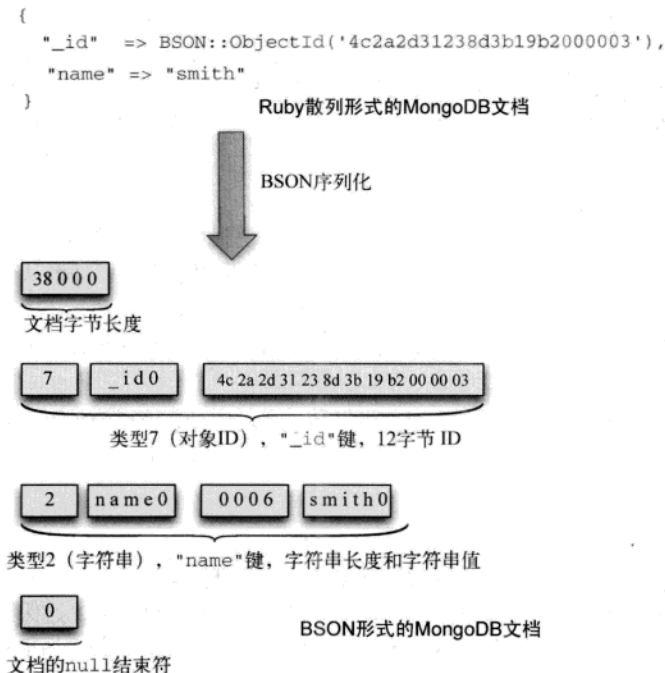
图3-2 从Ruby转换为BSON
