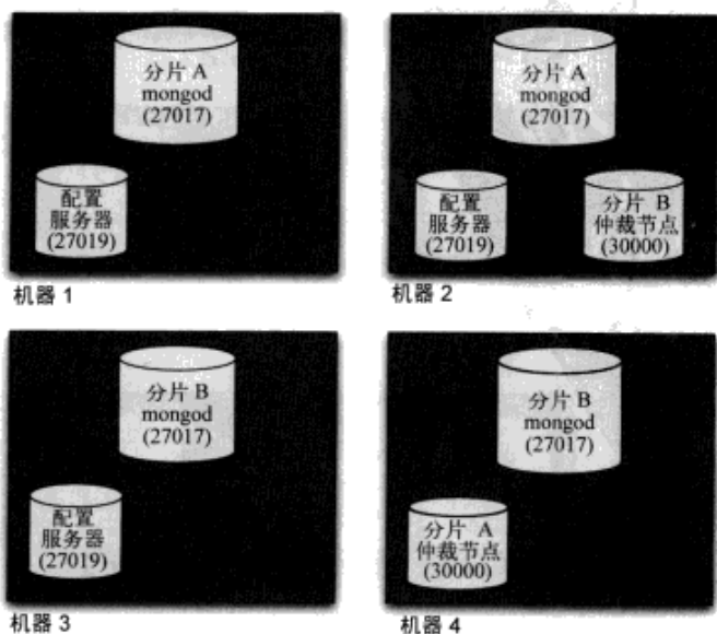
图9-4 部署在四台机器上的两分片集群
