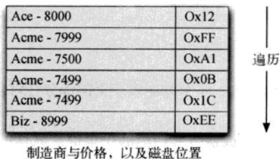
图7-3 复合键索引遍历
