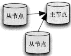
图1-3 副本集自动故障转移
