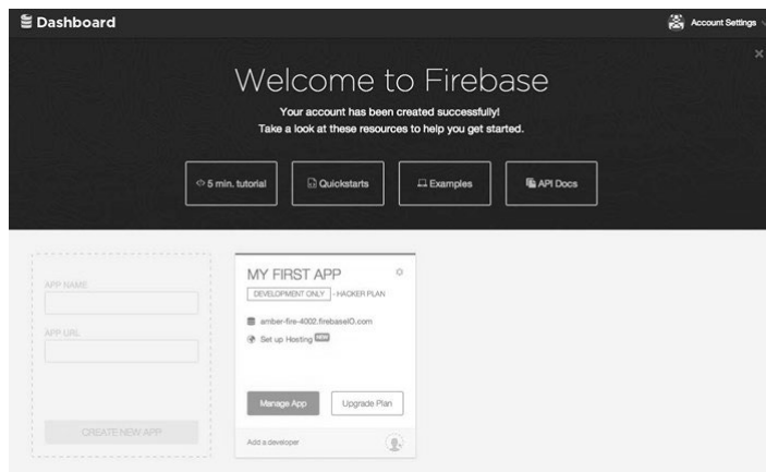
图18-23 注册过程
