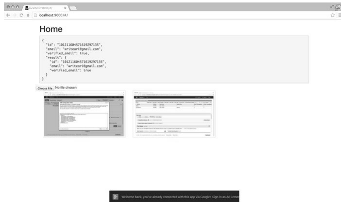
图18-17 图像清单
