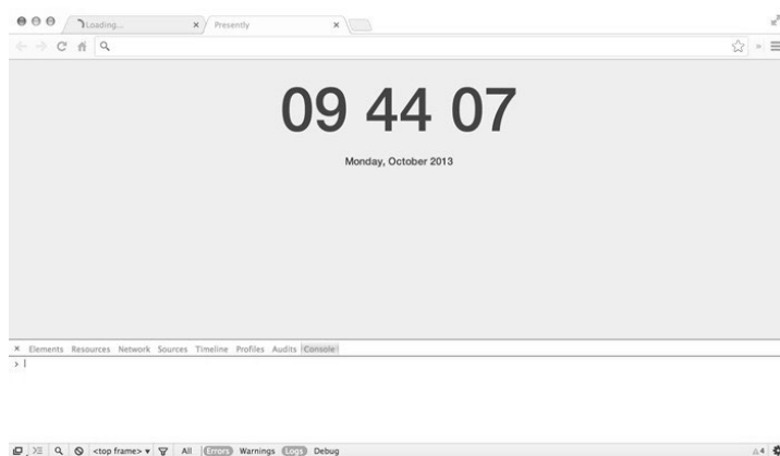
图31-6 完整的日期
