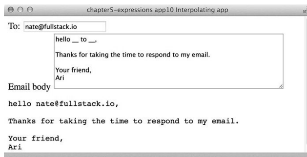
图6-1 插值文本
