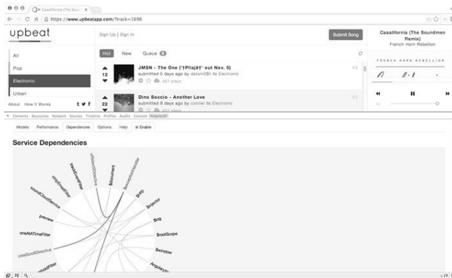
图33-4 依赖图表
