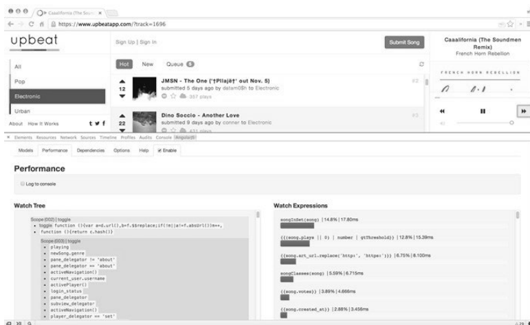
图33-3 性能检查器
