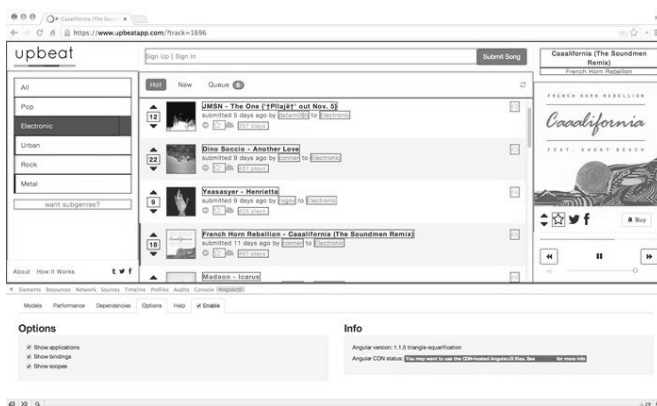
图33-5 选项面板
