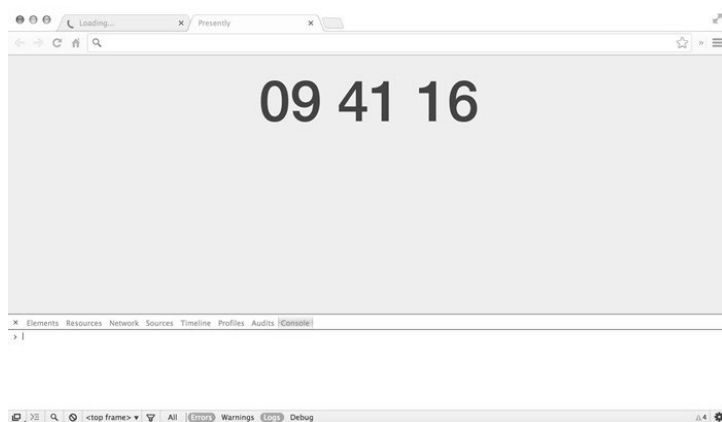
图31-5 第一个界面
