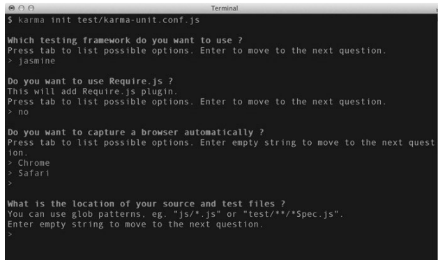
图19-2 Karma初始化
