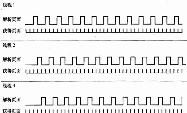
图 A-2 三个并发线程
