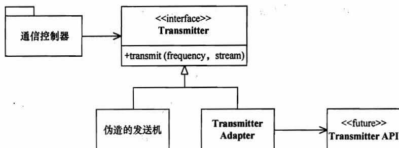
图 8-2 对发送器的预测
