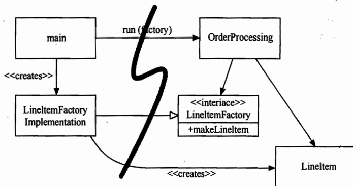
图 11-2 使用工厂分离构造过程
