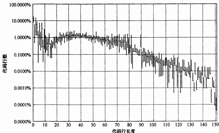
图 5-2 Java 程序代码行长度分布
