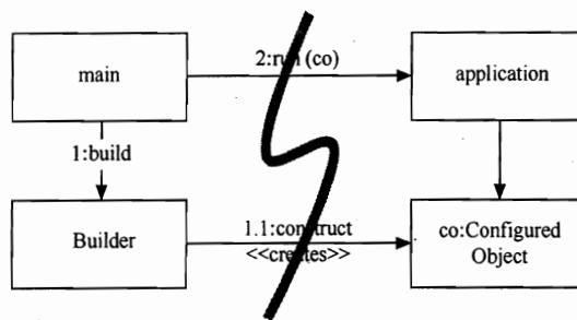
图 11-1 将构造分解到 main() 中
