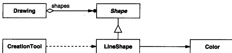
c) 类关系
