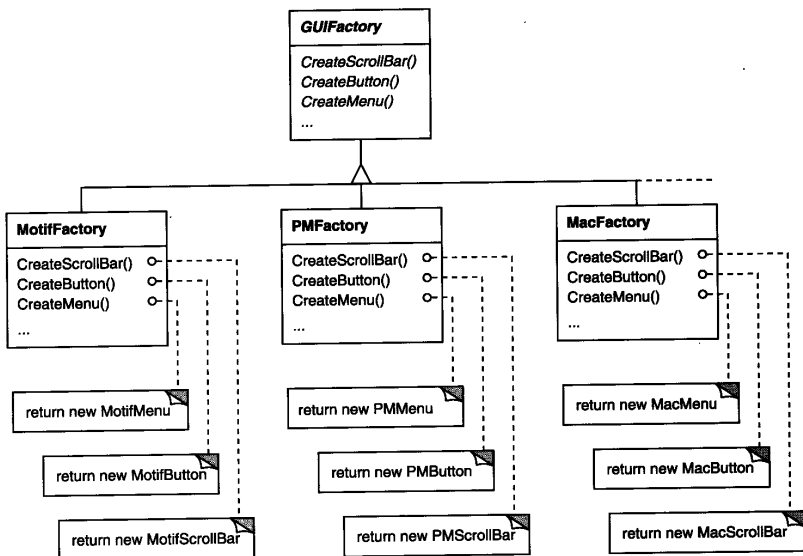
图 2-9 GUIFactory 类层次
