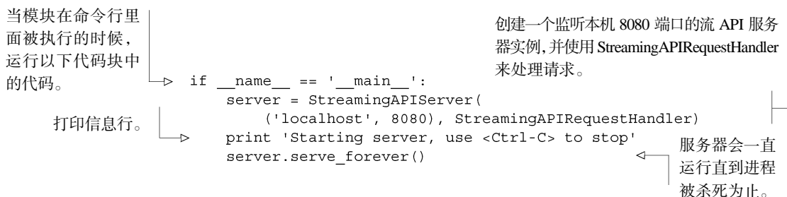
代码清单 8-10 启动并运行 HTTP 流服务器的代码
