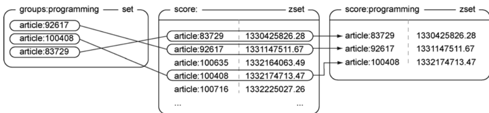
图 1-12 对集合 groups:programming 和有序集合 score: 进行交集计算得出了新的有序集合 score:programming ，它包含了所有同时存在于集合 groups:programming 和有序集合 score: 的成员。因为集合 groups:programming 的所有成员的分值都被视为是 1，而有序集合 score: 的所有成员的分值都大于 1，并且这次交集计算挑选的分值为相同成员中的最大分值，所以有序集合 score:programming 的成员的分值实际上是由有序集合 score: 的成员的的分值来决定的
