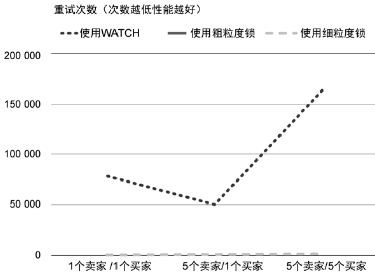
图 6-4 在 60 秒内因为购买商品而引发的重试次数。因为两种锁实现都不会引发重试，而记录细粒度锁数据的线条正好覆盖住了记录粗粒度锁数据的线条，因此我们在图中只会看见记录细粒度锁数据的线条，而看不见记录粗粒度锁数据的线条
