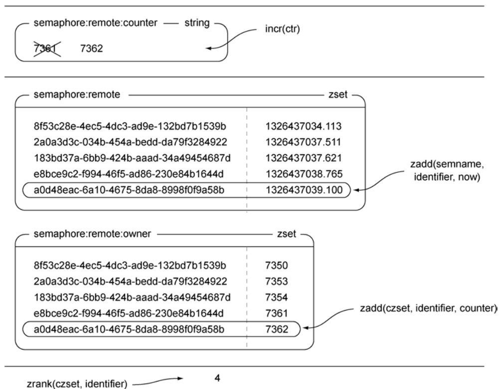
图 6-8 acquire_fair_semaphore() 函数的调用序列
