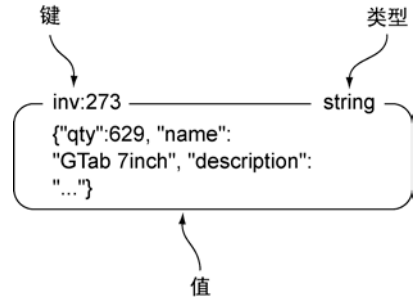
图 2-1 一个被缓存的数据行，这个数据行包含了在线售卖商品的信息
