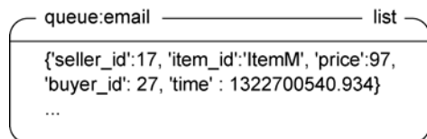
图 6-9 一个使用列表结构实现的先进先出队列
