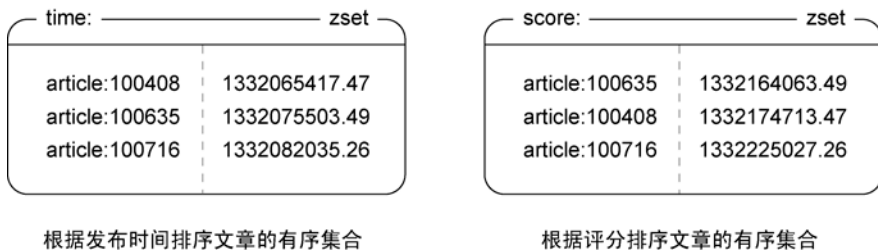
图 1-9 两个有序集合分别记录了根据发布时间排序的文章和根据评分排序的文章
