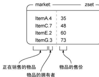
图 4-3 一个基本的商品买卖市场，其中用户 4 正在销售商品 ItemA，售价为 35 块钱
