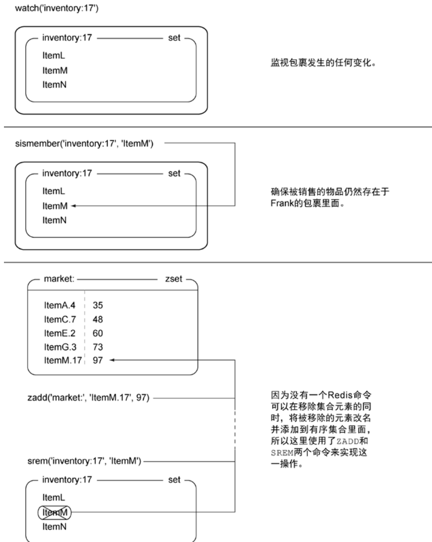
图 4-4 list_item(conn, "ItemM", 17, 97) 的执行过程
