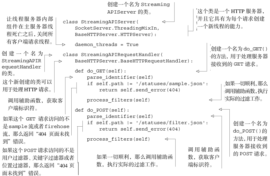
代码清单 8-9 HTTP 流服务器及其请求处理器
