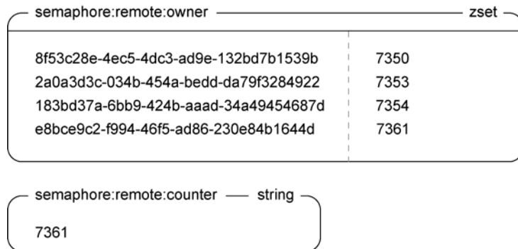
图 6-7 公平信号量的数据结构示例
