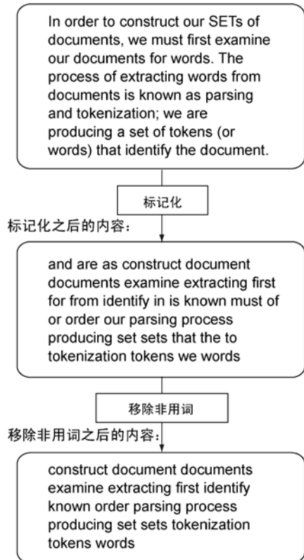
图 7-2 将本节的一部分原文标记化为多个单词,并移除其中的非用词
