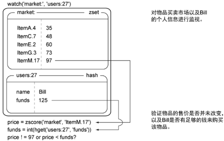
图 4-5 在购买指定商品之前，程序必须对商品买卖市场以及买家的个人信息进行监视，检查指定商品是否仍然存在，以及买家是否有足够的钱来购买该商品
