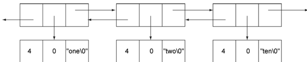
图 9-1 Redis 存储长列表的方式
