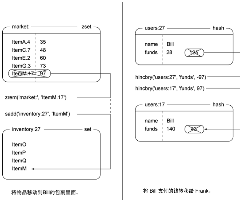
图 4-6 商品购买操作的执行流程如下：程序首先需要将买家支付的钱转移给卖家，然后从商品买卖市场里面移除被售出的商品，最后将该商品添加到买家的包裹里面
