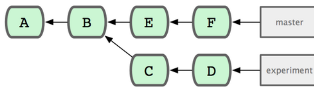
图 6.1: 范围选择的提交历史实例
