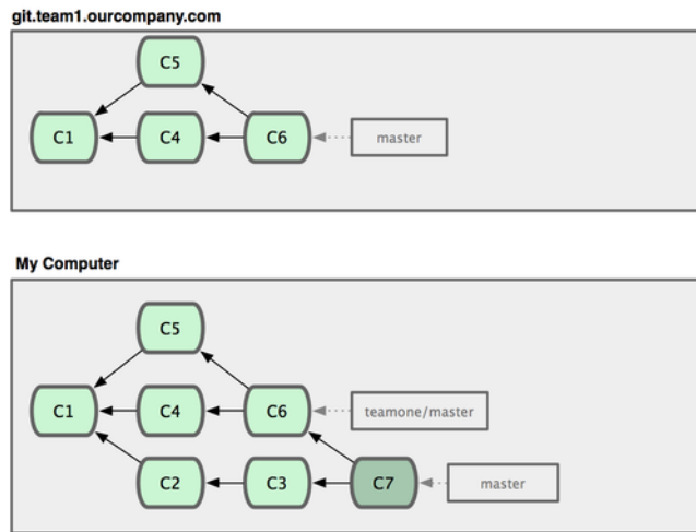
图 3.37：获取更多提交，并入你的开发进程。
