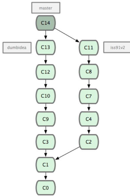
图 3.21: 合并了 dumbidea 和 iss91v2 以后的历史。
