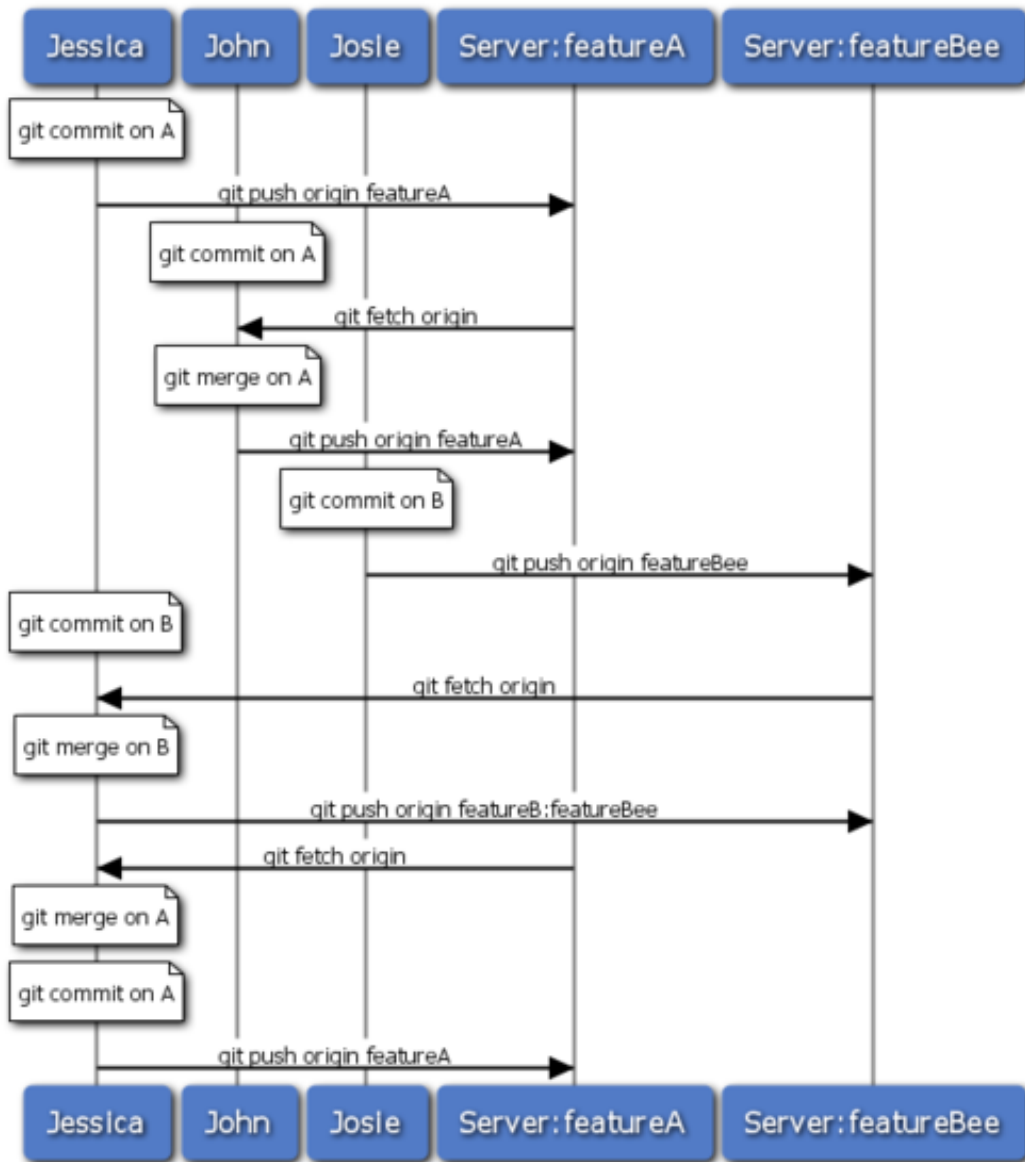
图 5.15: 团队间协作工作流程基本时序
