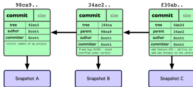
图 3.2: 多次提交后的 Git 对象数据
