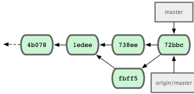
图 5.6: 推送后 John 的仓库历史
