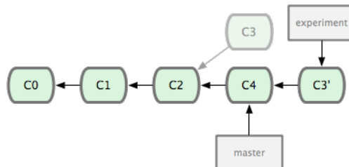
图 3.29: 把 C3 里产生的改变衍合到 C4 中。
