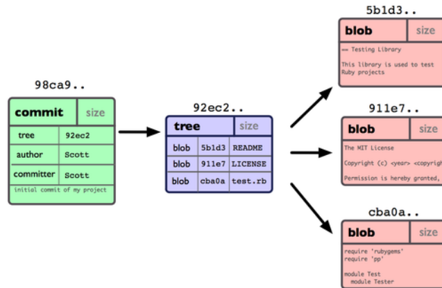
图 3.1: 一次提交后仓库里的数据
