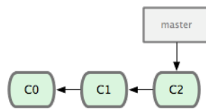
图 3.10：一部分简短的提交历史
