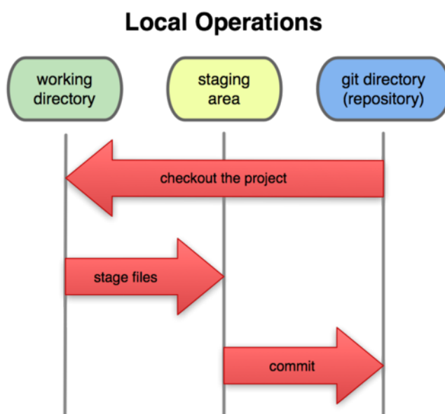
图 1.6: 工作目录，暂存区域和 git 目录
