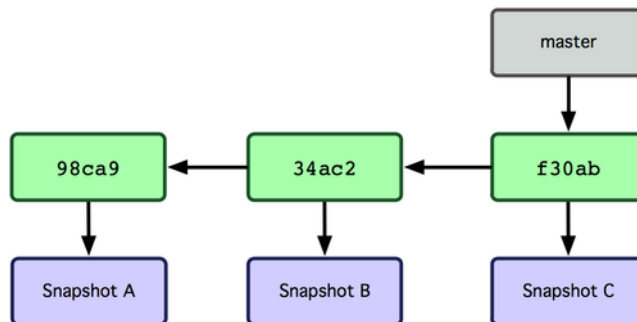
图 3.3: 指向提交数据历史的分支
