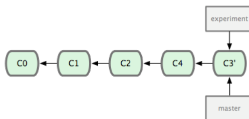
图 3.30: master 分支的快进。
