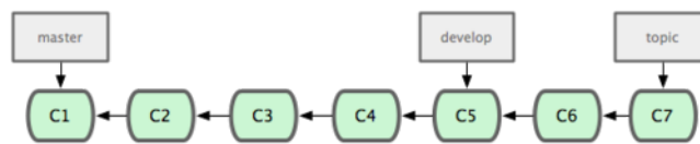
图 3.18: 稳定分支总是比较老旧。
