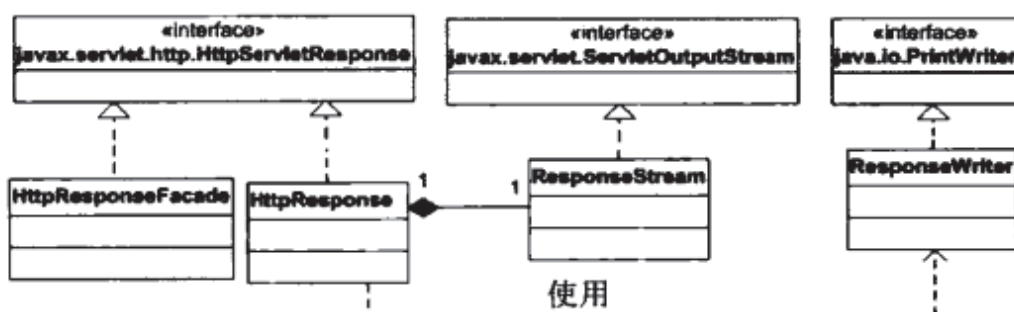
图 3-3 HttpResponse 及其相关类的 UML 类图
