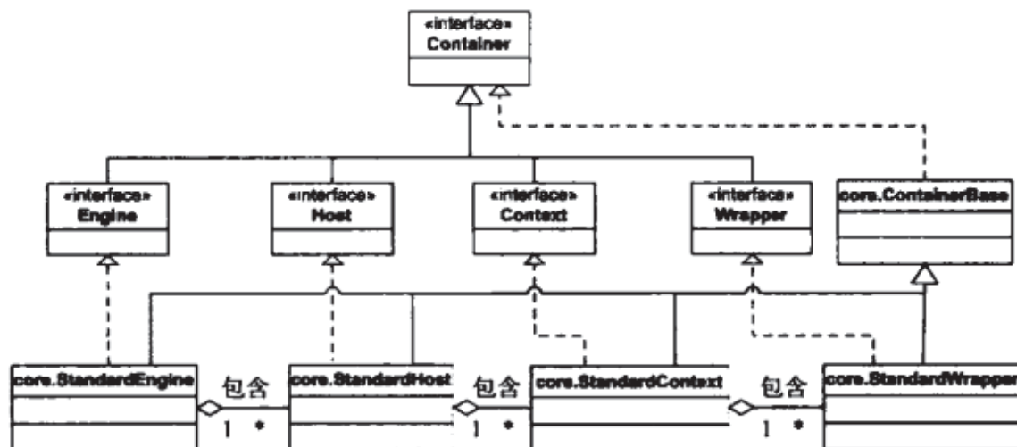
图 5-1 Container 接口及其相关类的 UML 类图
