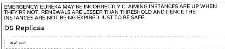
图 4-10 Eureka Server 自我保护模式界面
