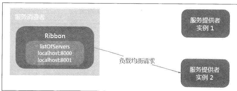
图 5-3 脱离 Eureka 使用 Ribbon 架构图
