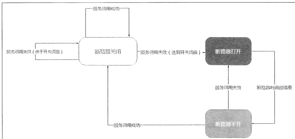
图 7-2 断路器状态转换图
