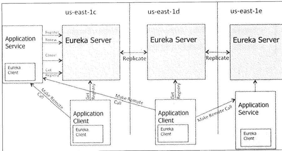
图 4-3 Eureka 架构图
