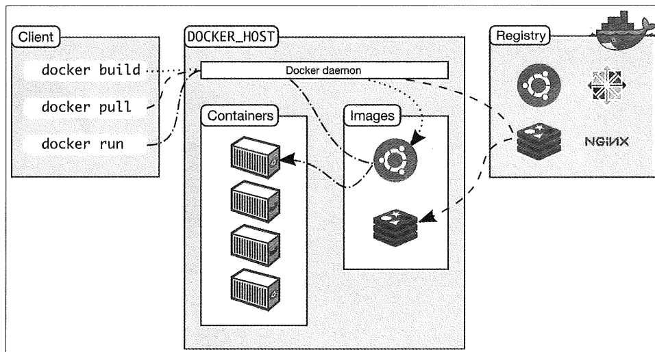
图 12-1 Docker 架构图
