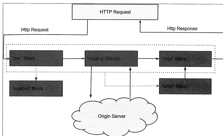
图 8-5 Zuul 请求的生命周期
