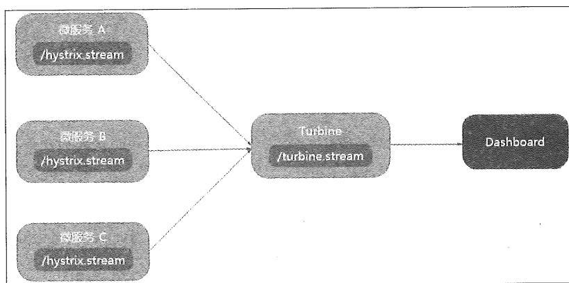
图 7-6 微服务引入 Turbine 架构图
