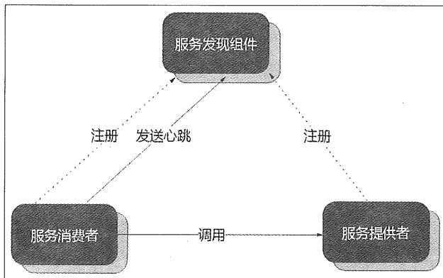
图 4-1 服务发现架构图
