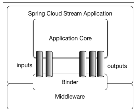
图5. Spring Cloud Stream应用
