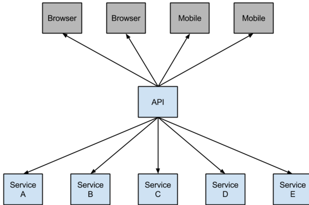
图7.微服务图
