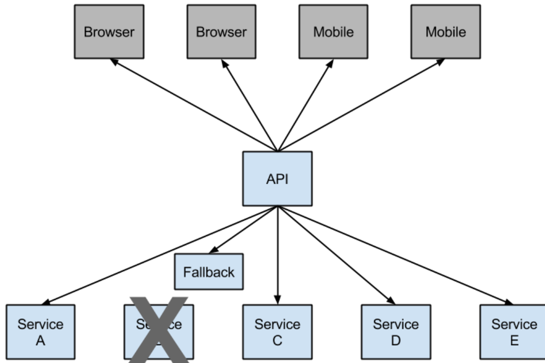
图2. Hystrix回退防止级联故障
