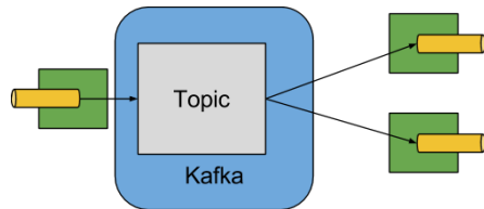
图13. Kafka Binder
