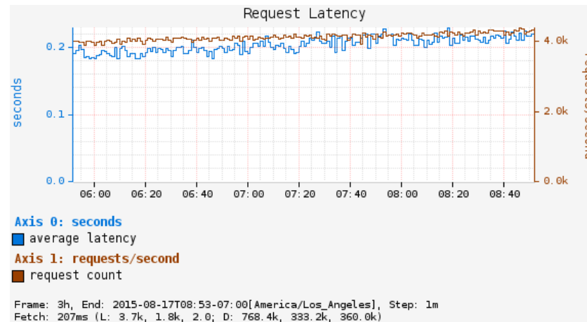
图4. 请求延迟
