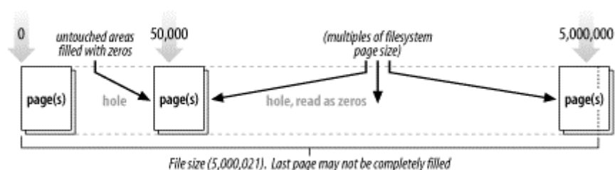
图 3-8 有两个空洞的磁盘文件
