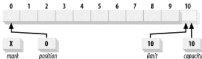
图 2-2. 新创建的 ByteBuffer
