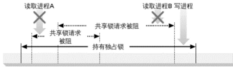
图 1-8. 独占锁阻断共享锁请求
