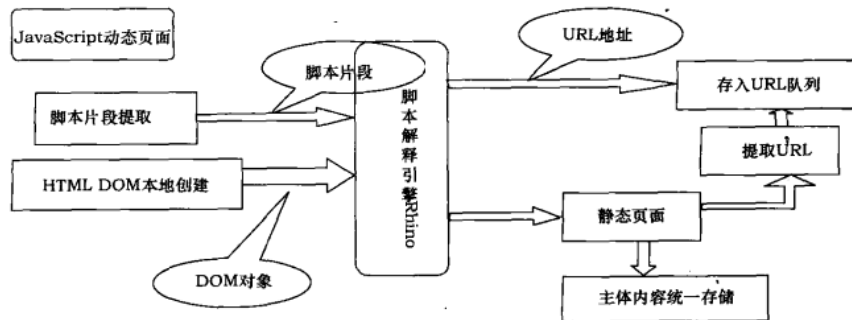
图 4.2 基于 Rhino 实现 JavaScript 动态页面解析的过程
