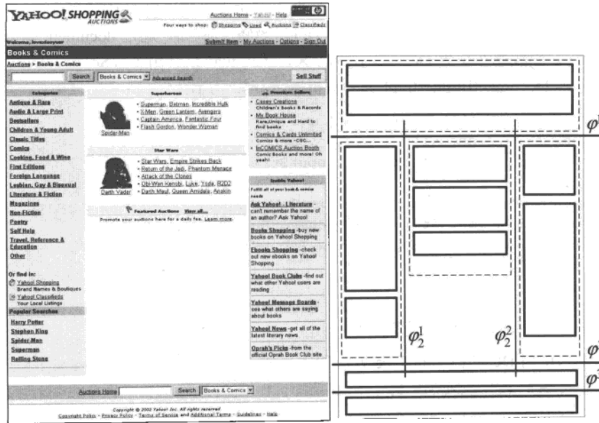
图 7.10 从网页到布局特征
