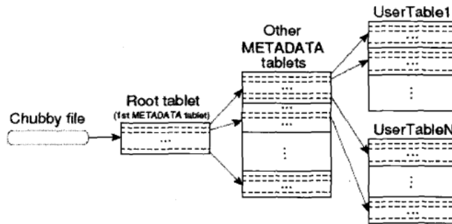
图 2.13 BT 的 B+树的体系结构
