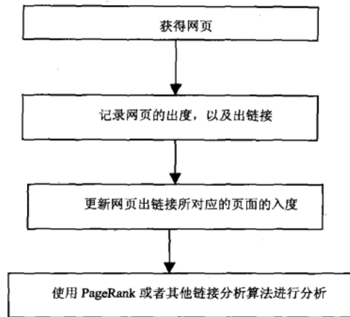
图 8.3 链接分析过程
