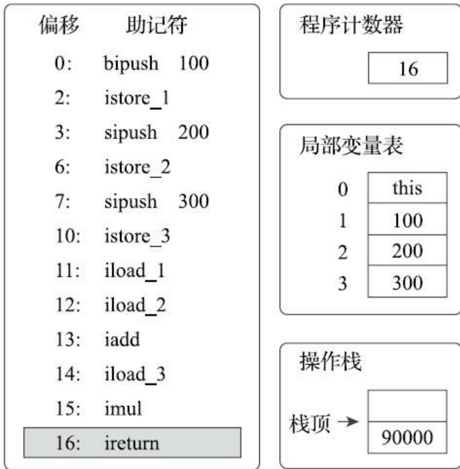
图8-11 执行偏移地址为16的指令的情况
