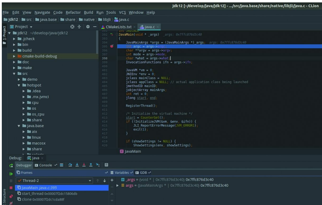
图1-12 在CLion中创建HotSpot项目（3）
