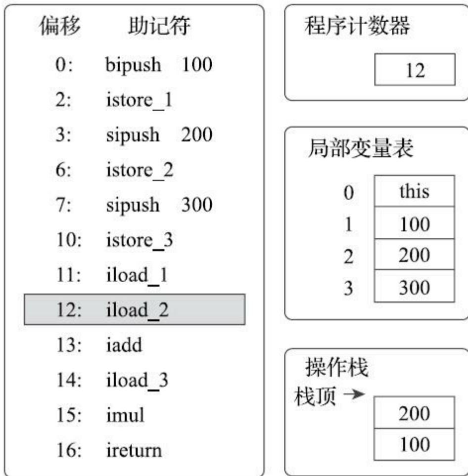
图8-8 执行偏移地址为12的指令的情况
