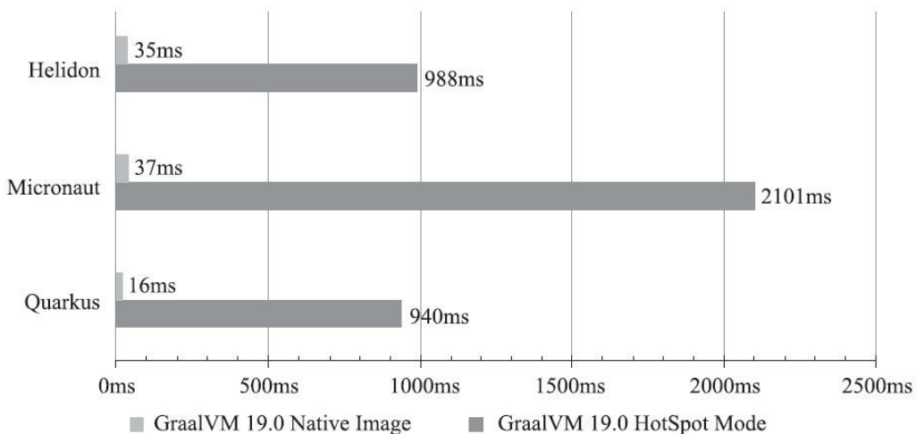
图1-6 启动时间对比
