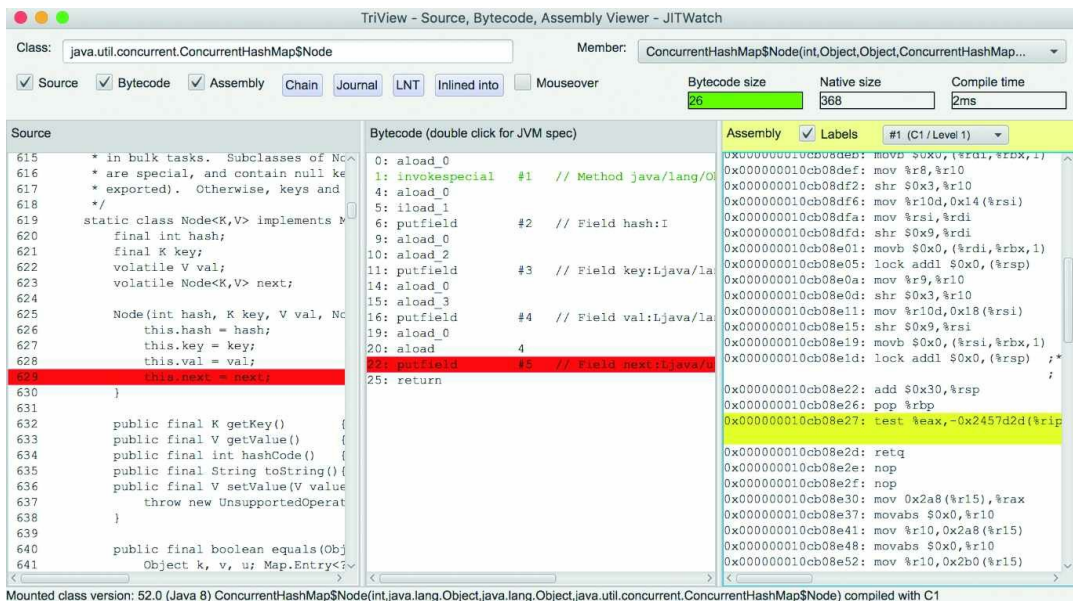
图4-29 查看方法代码
