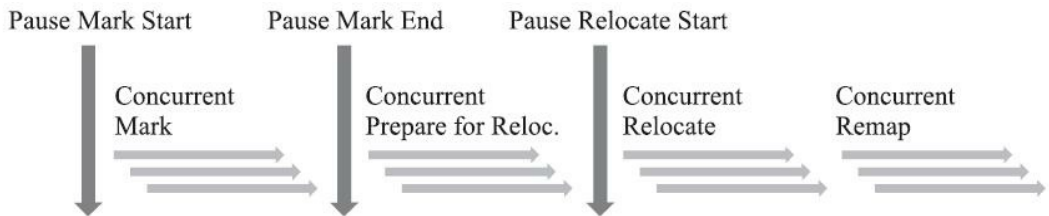
图3-22 ZGC运作过程
