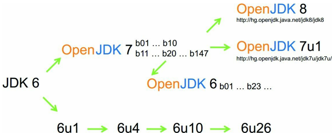
图1-8 OpenJDK版本之间的关系
