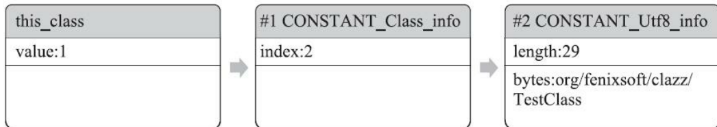
图6-6 类索引查找全限定名的过程
