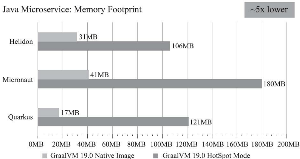
图1-5 内存占用对比
