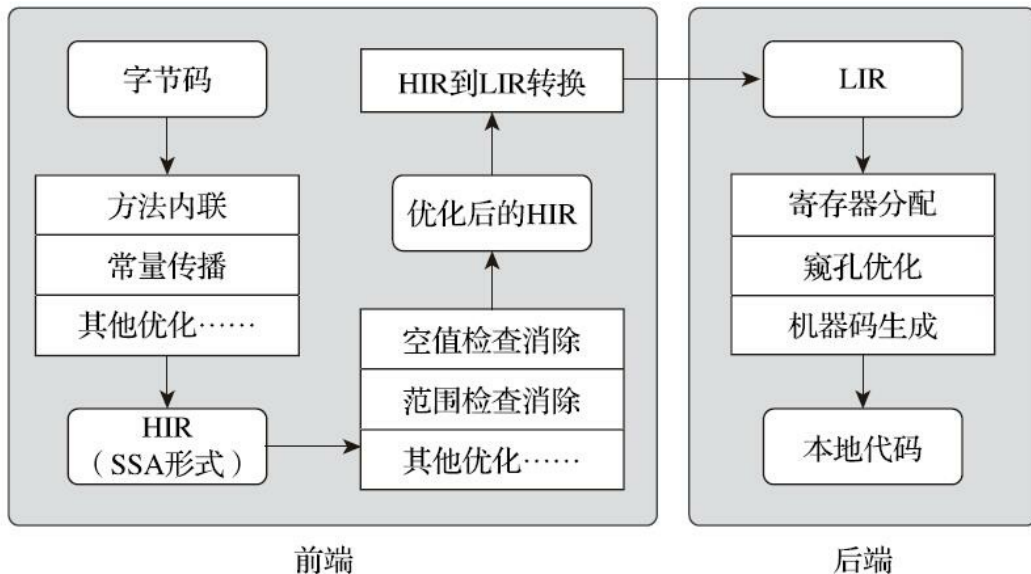
图11-5 Client Compiler架构
