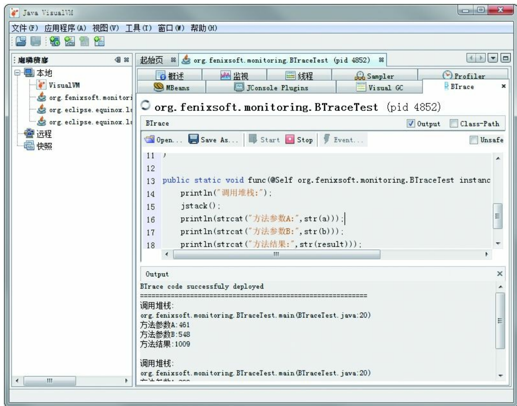
图4-23 BTrace跟踪结果
