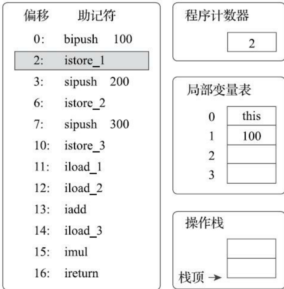
图8-6 执行偏移地址为1的指令的情况
