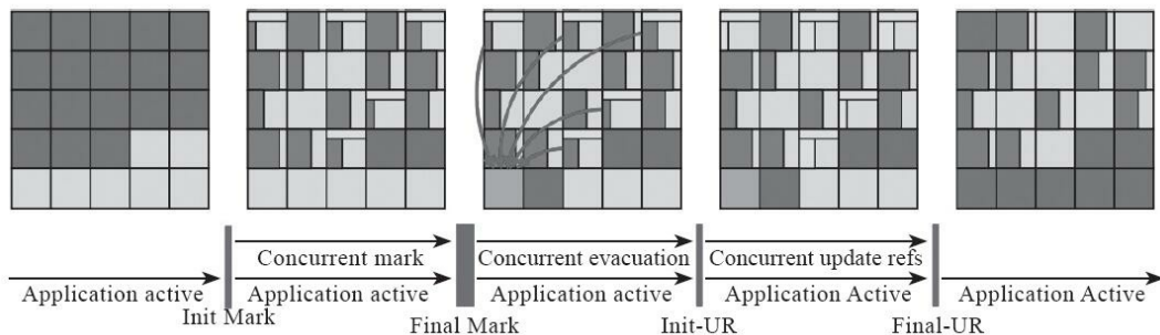
图3-16 Shenandoah收集器的工作过程
