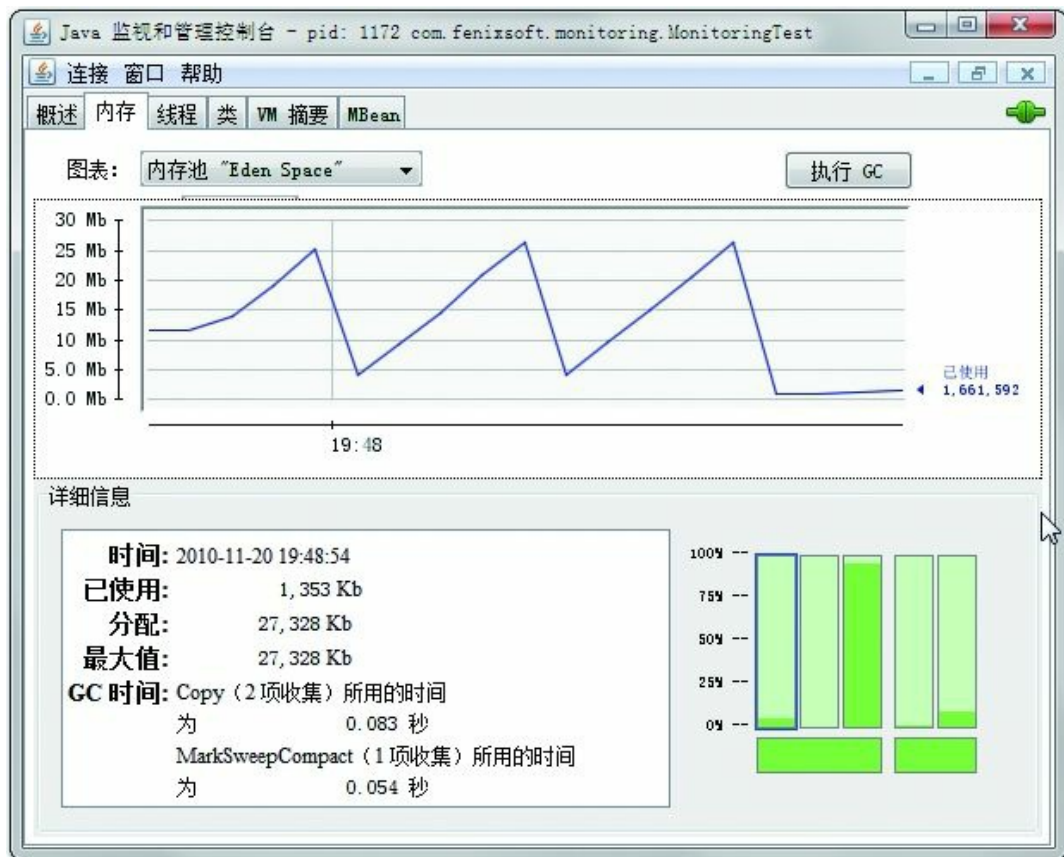
图4-12 Eden区内内存变化状况
