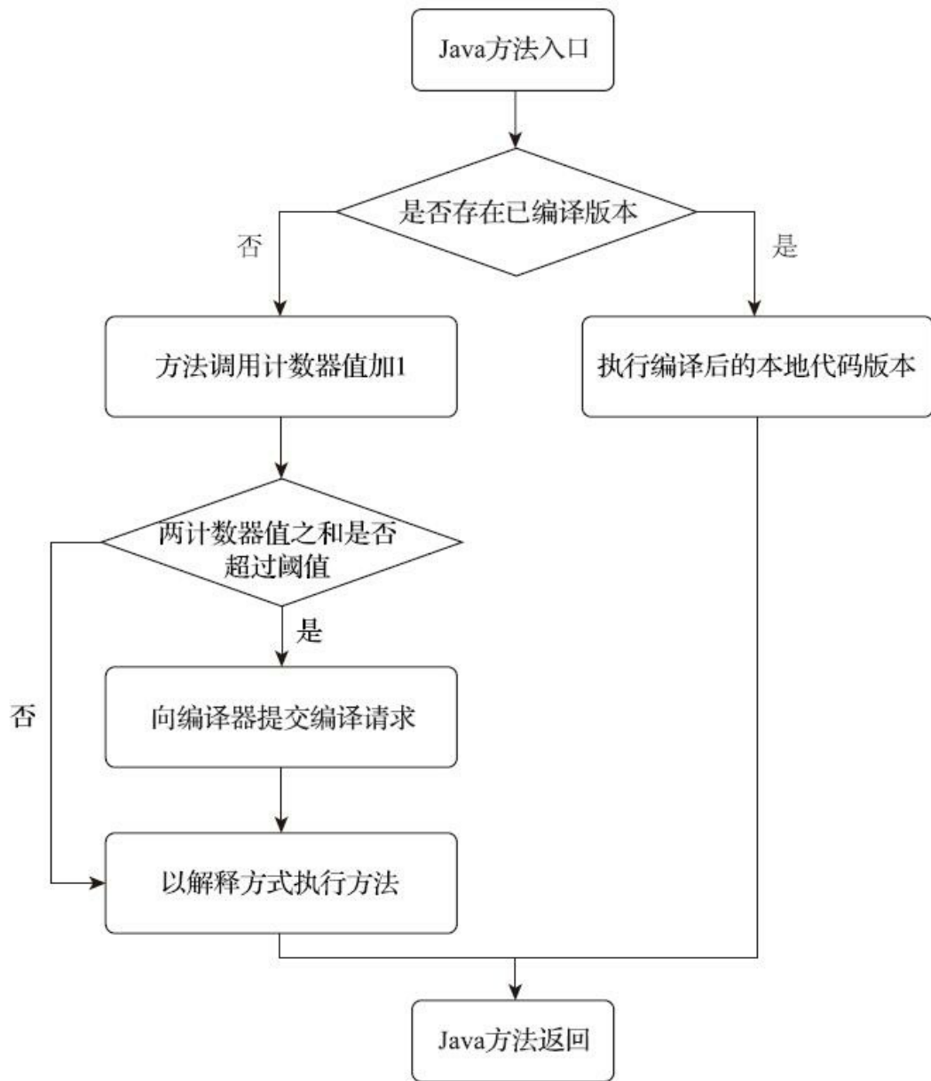
图11-3 方法调用计数器触发即时编译
