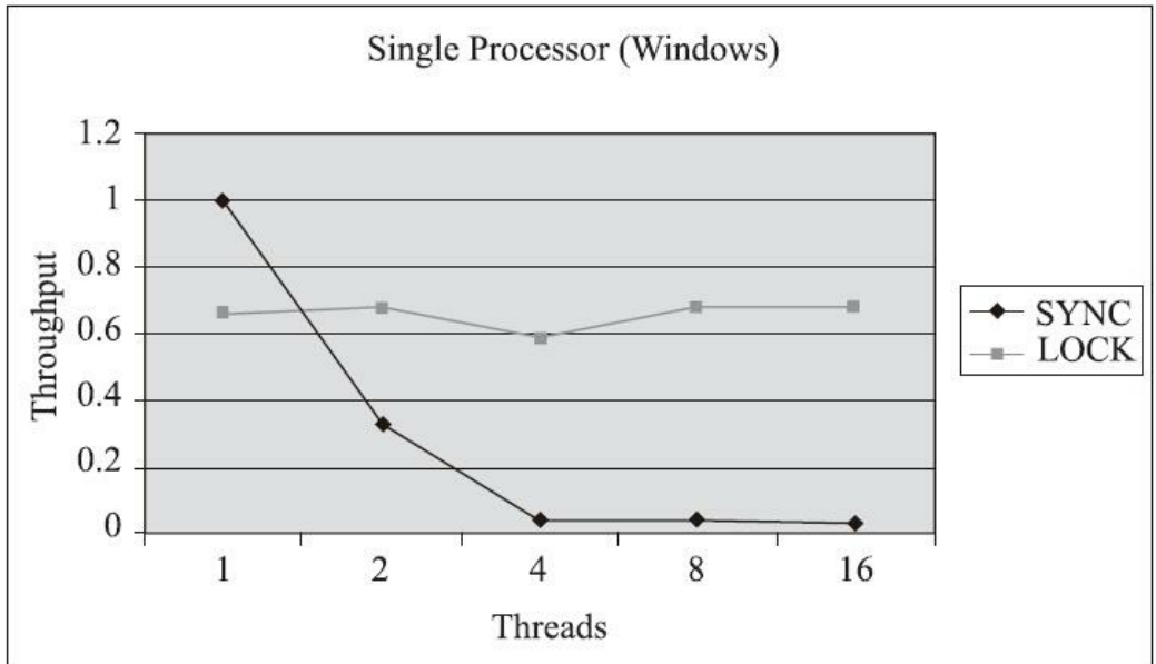
图13-1 JDK 5、单核处理器下两种锁的吞吐量对比
