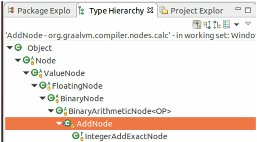
图11-19 节点继承关系
