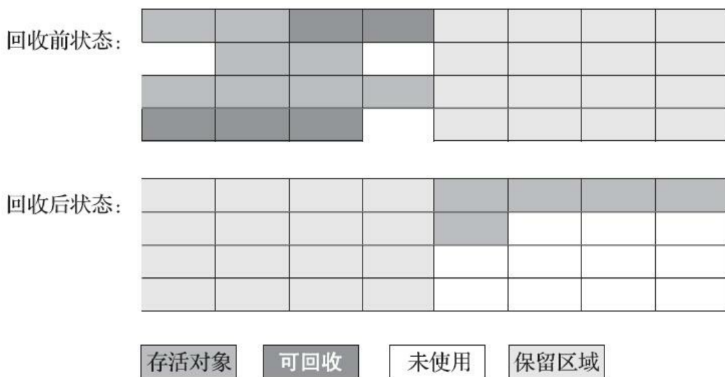
图3-3 标记-复制算法示意图
