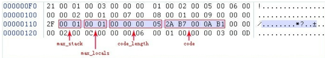
图6-10 Code属性结构实例
