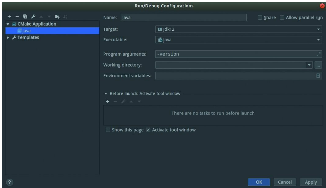
图1-11 在NetBeans中创建HotSpot项目（2）
