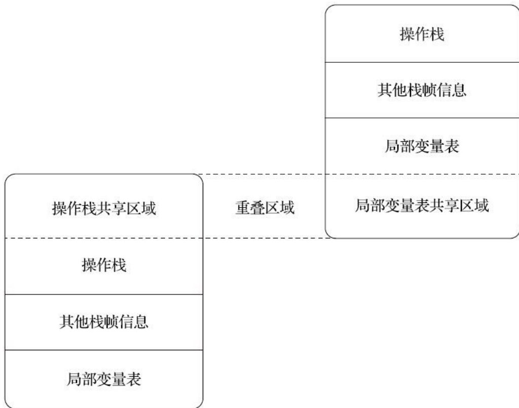
图8-2 两个栈帧之间的数据共享
