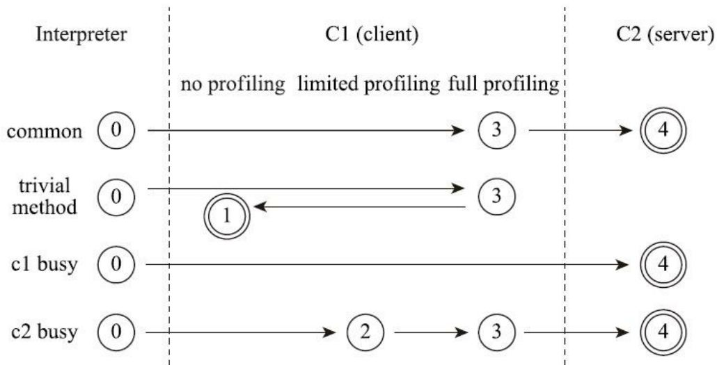
图11-2 分层编译的交互关系 [3]
