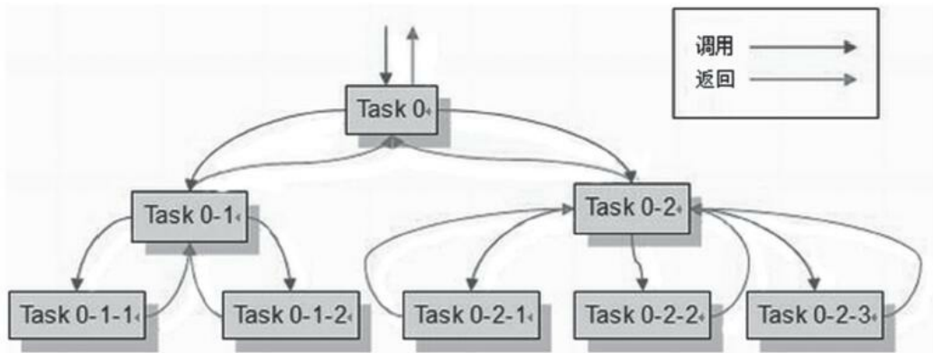
图B-2 Fork/Join模式示意图 [4]
