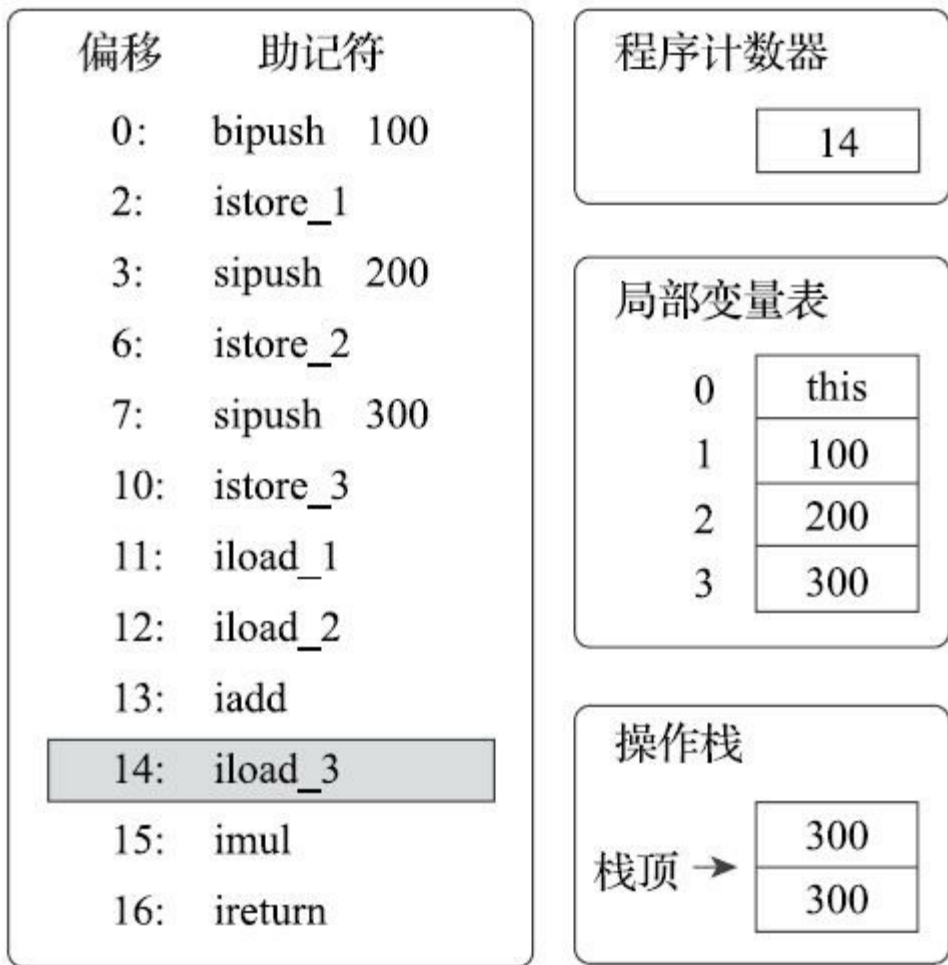
图8-10 执行偏移地址为14的指令的情况
