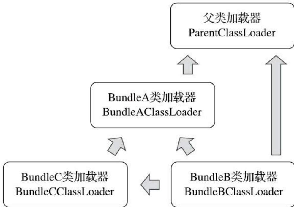
图9-2 OSGi的类加载器架构
