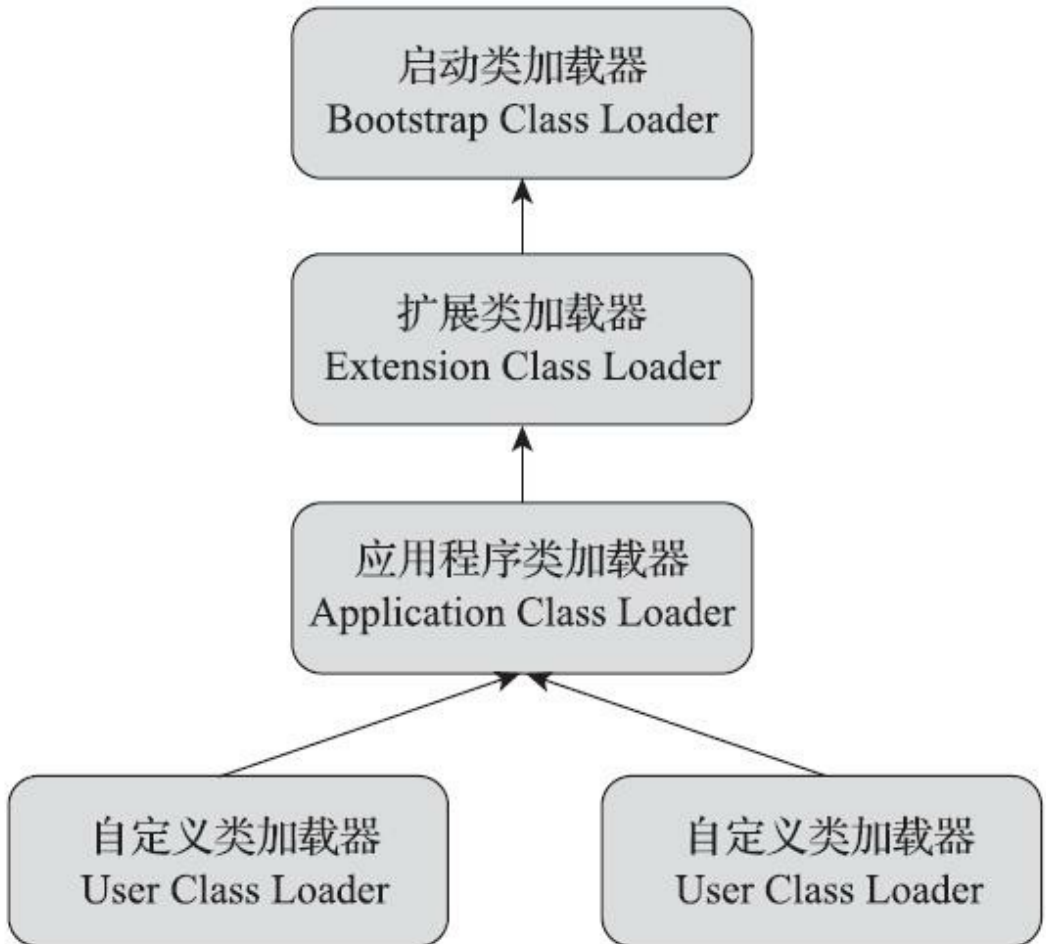
图7-2 类加载器双亲委派模型
