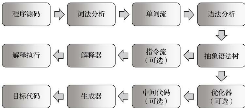
图8-4 编译过程
