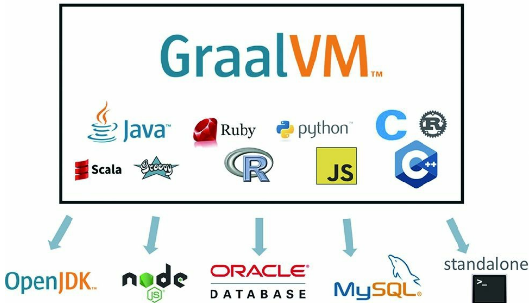
图1-4 Graal VM
