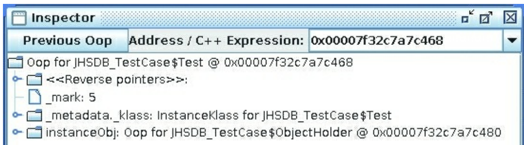
图4-8 JHSDB_TestCase$Test对象
