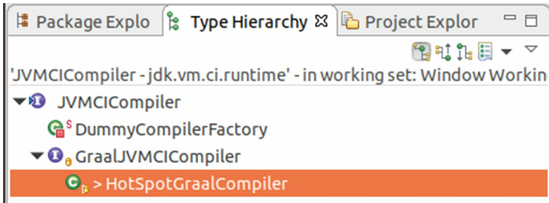
图11-12 JVMCI接口的继承关系
