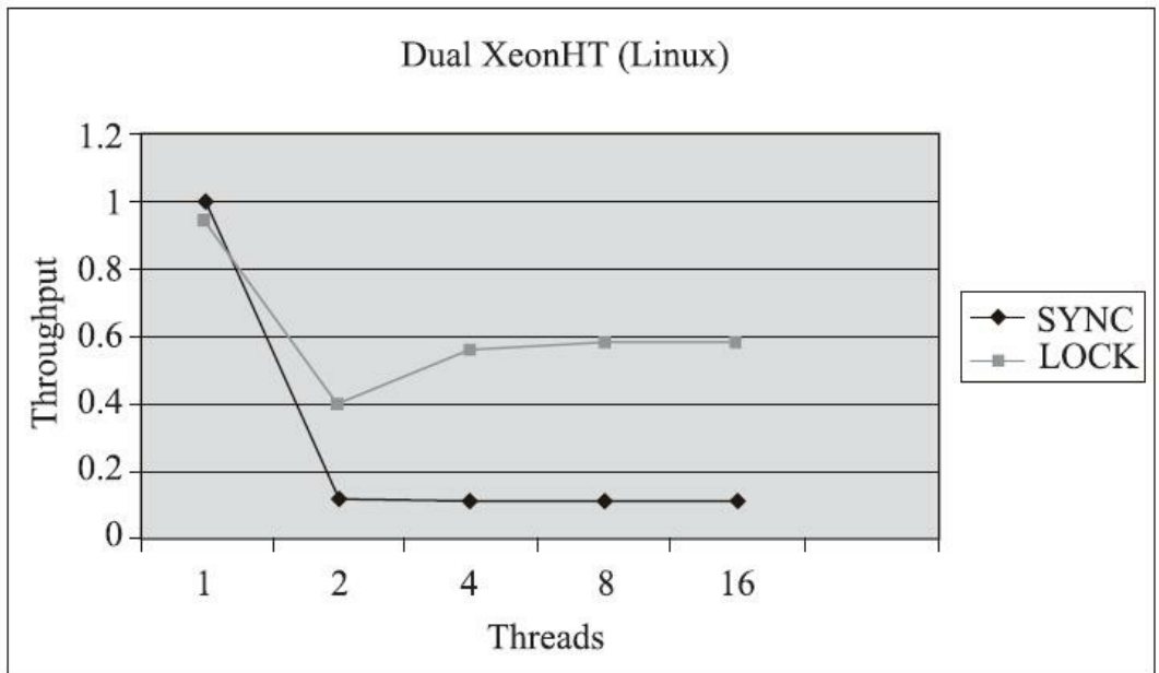
图13-2 JDK 5、双Xeon处理器下两种锁的吞吐量对比
