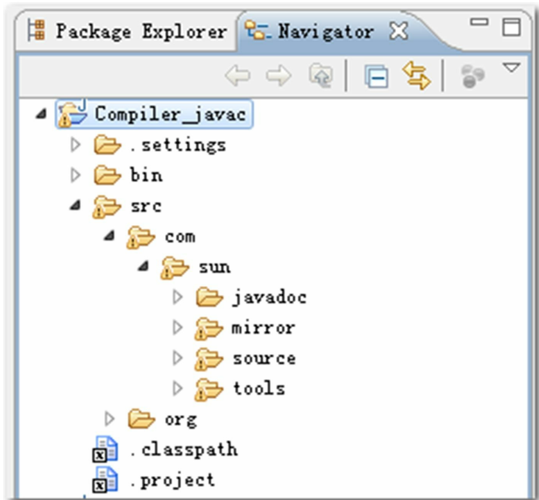
图10-1 Eclipse中的Javac工程
