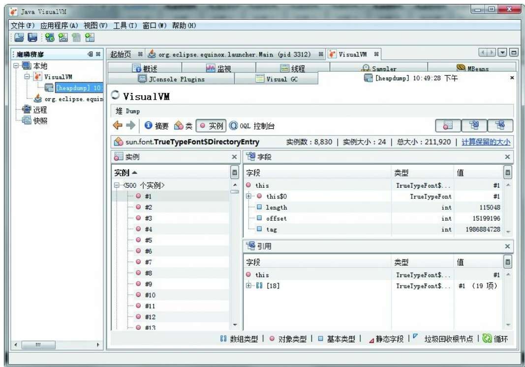
图4-20 浏览dump文件
