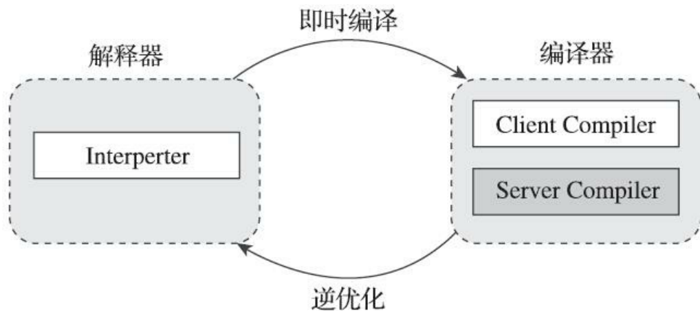
图11-1 解释器与编译器的交互
