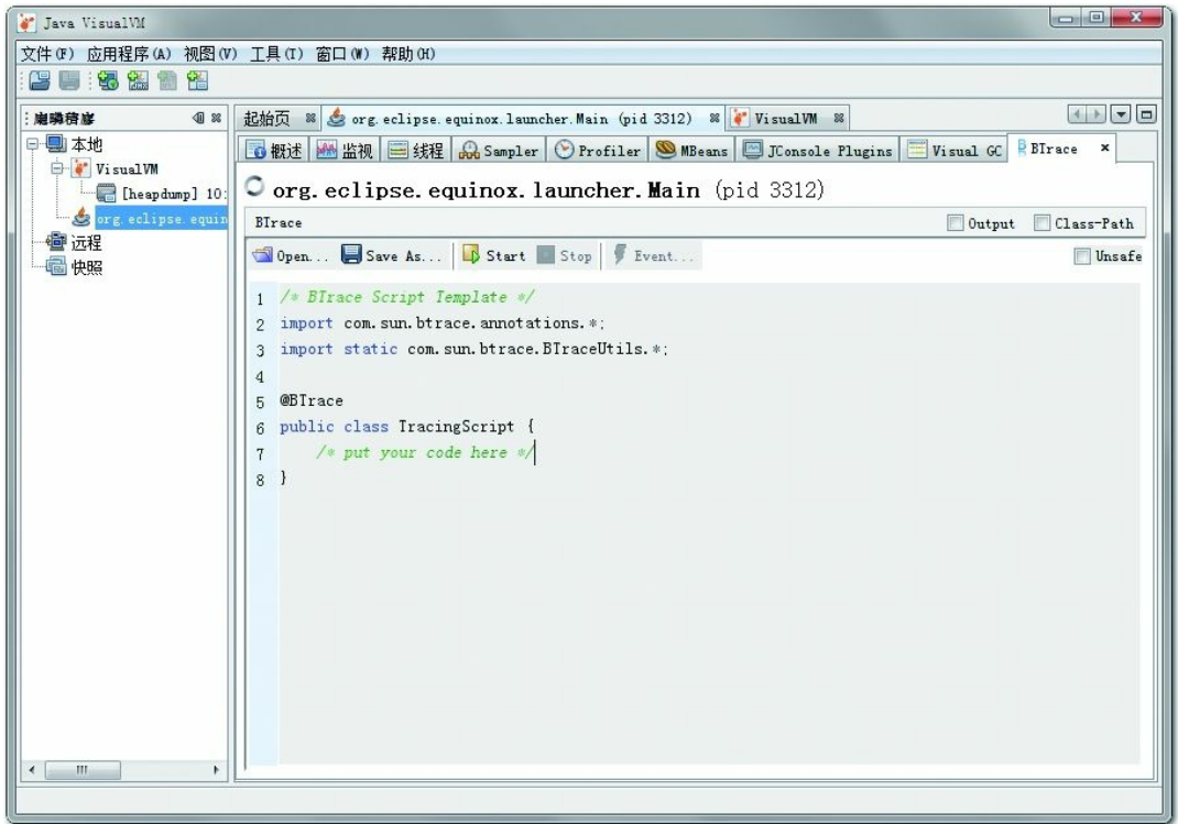
图4-22 BTrace动态跟踪
