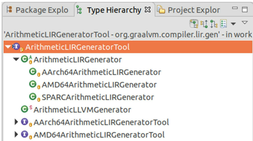
图11-21 Graal支持的目标平台生成器
