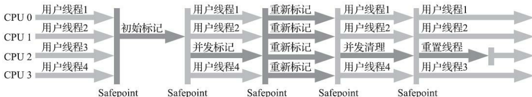
图3-11 Concurrent Mark Sweep收集器运行示意图
