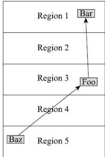
图3-15 Shenandoah收集器的连接矩阵示意图
