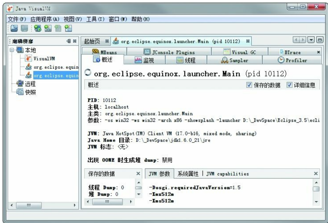
图4-19 VisualVM主界面
