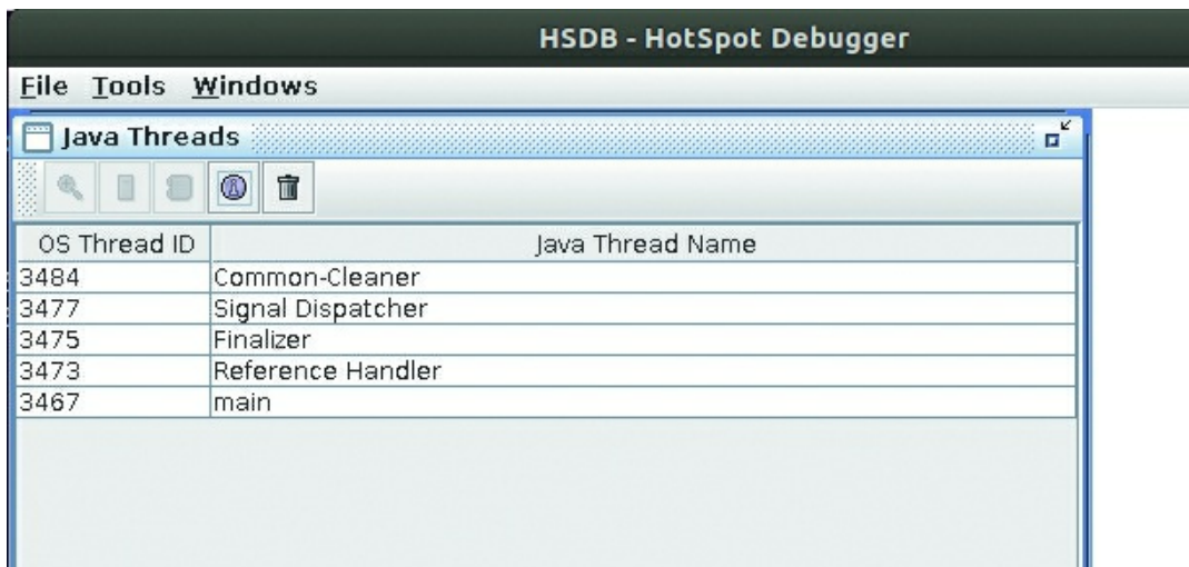
图4-4 JHSDB的界面
