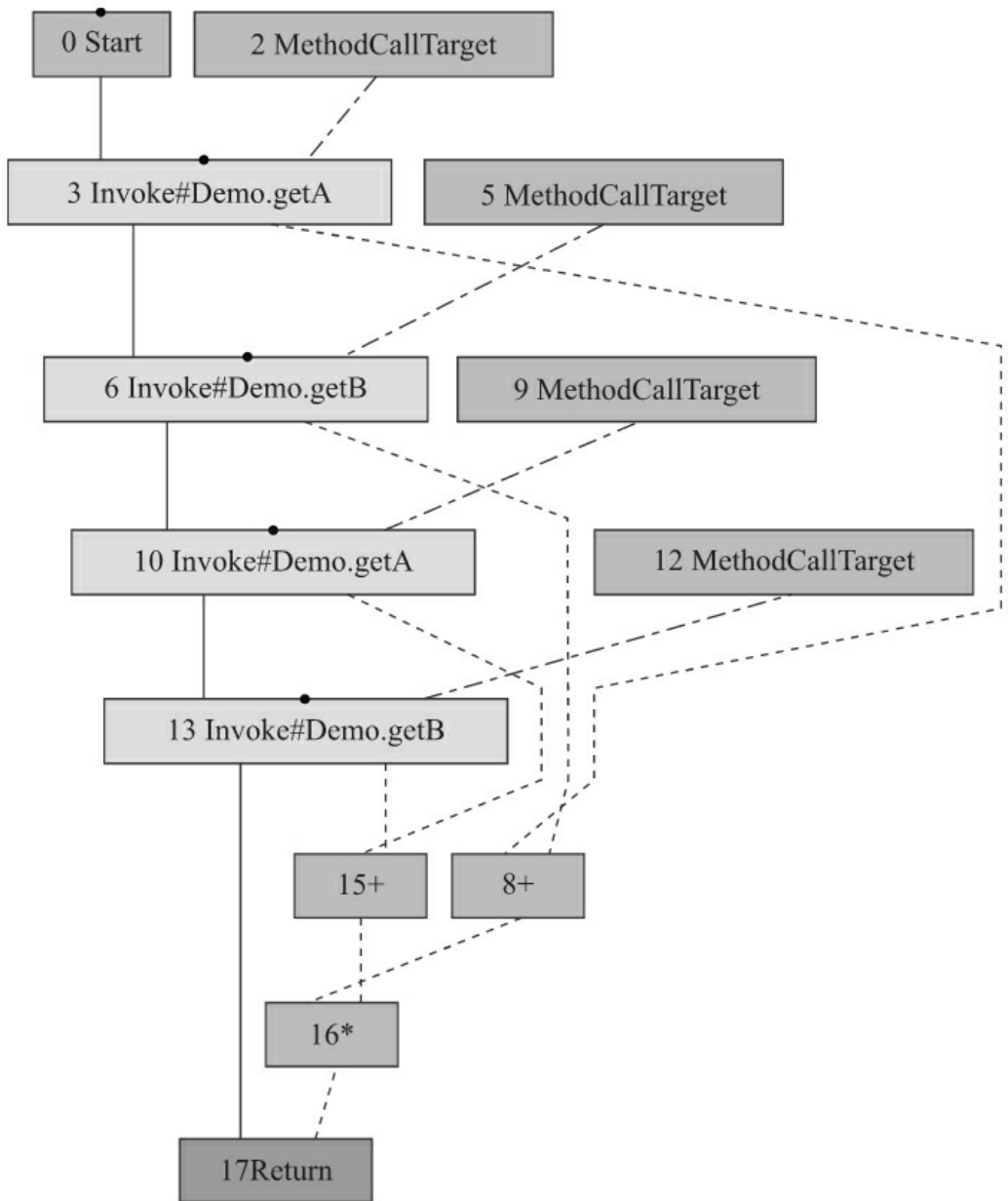
图11-17 构造理想图 (5)
