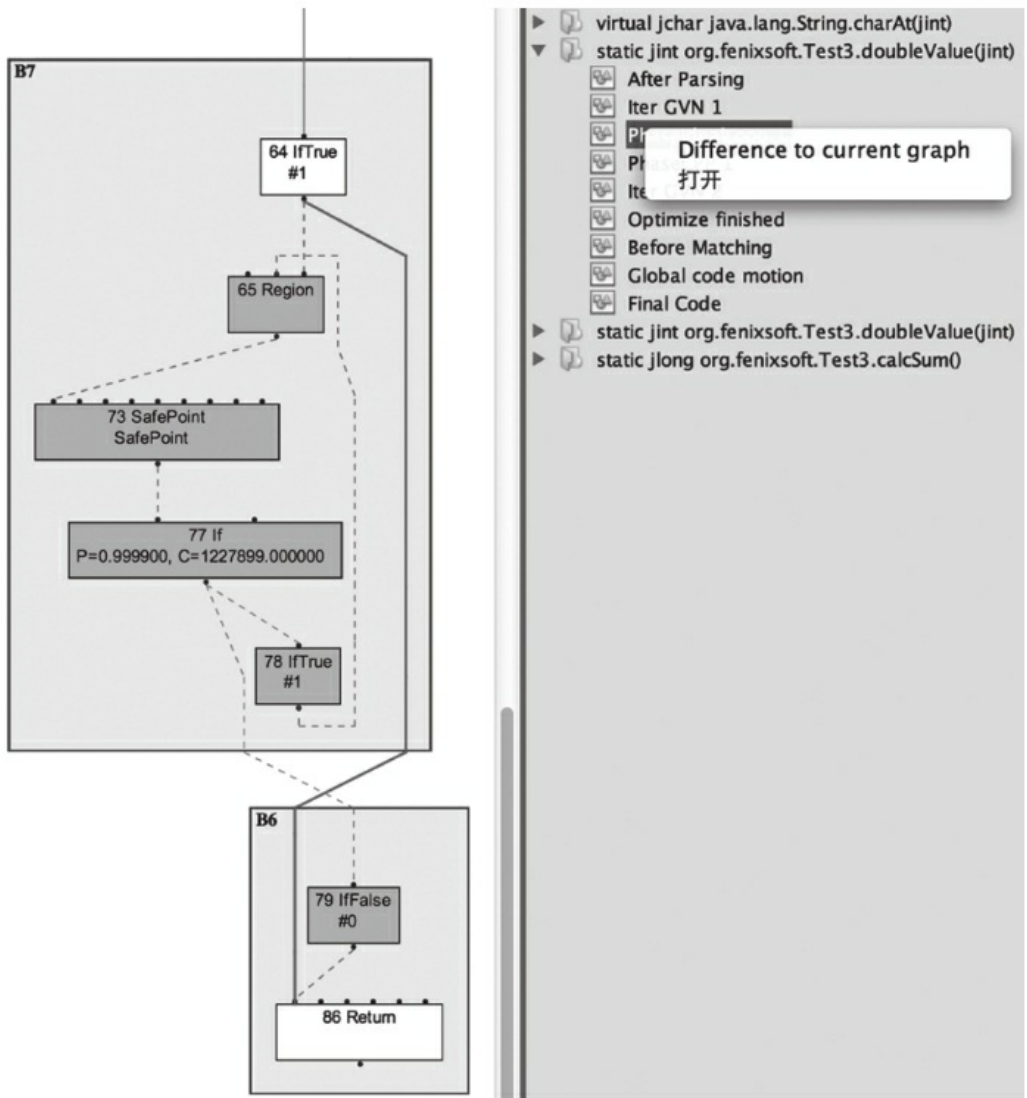
图11-9 基本块图示 (3)
