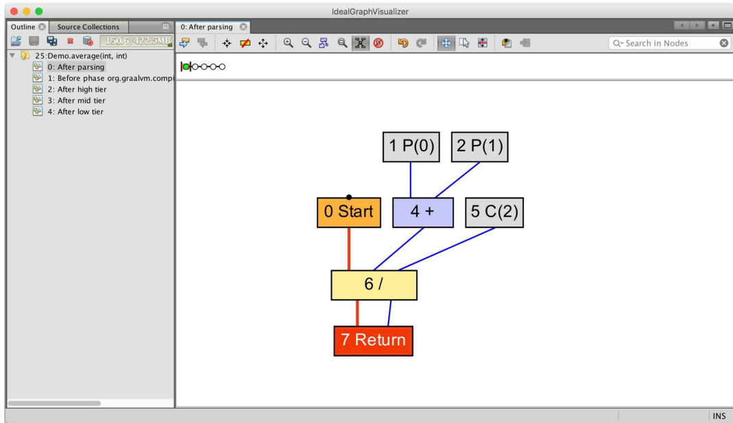
图11-15 构造理想图（3）
