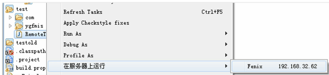
图9-4 JavaClassExecuter的使用
