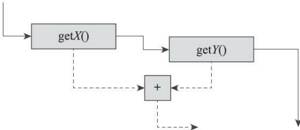
图11-14 构造理想图 (2)
