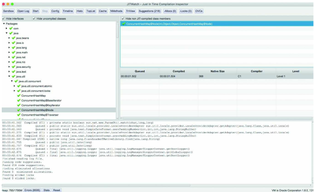
图4-28 JITWatch主界面
