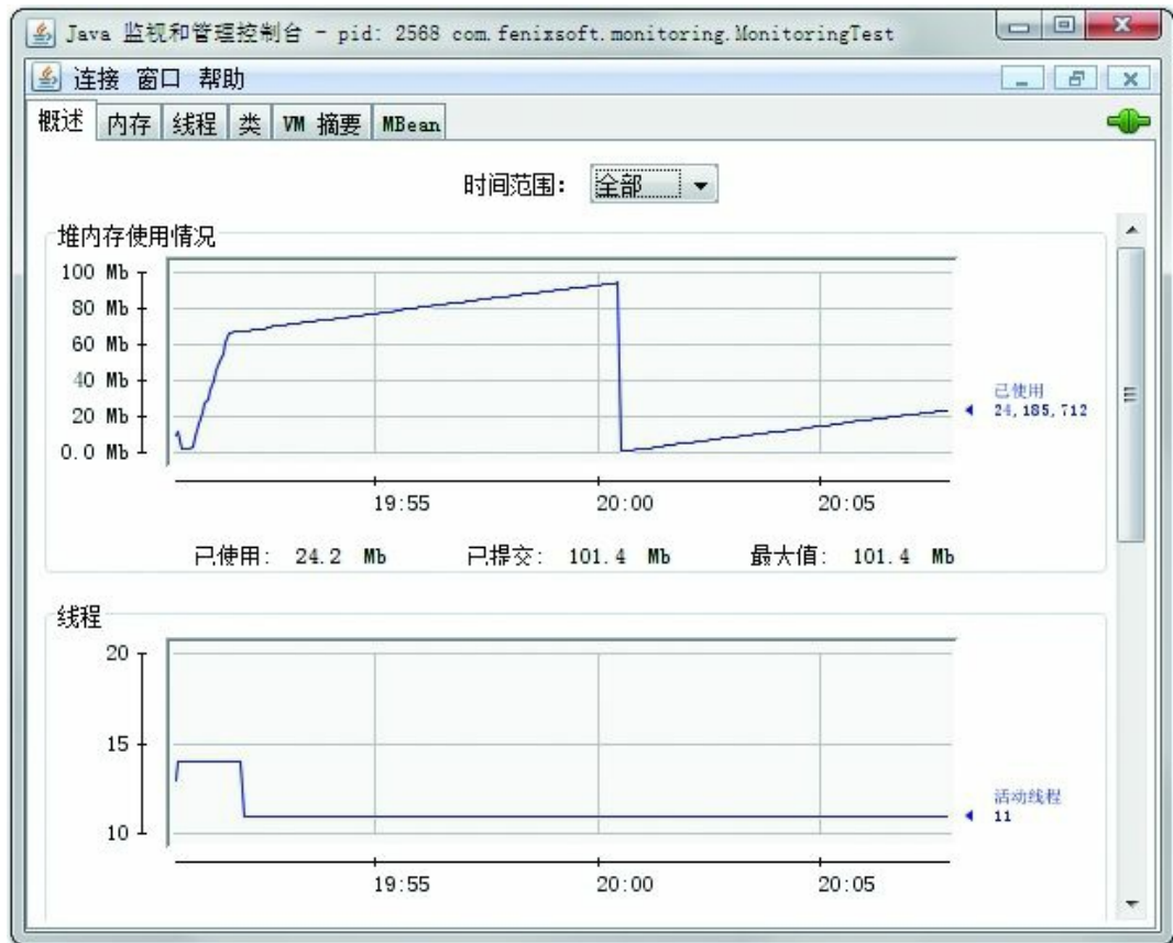
图4-11 JConsole主界面
