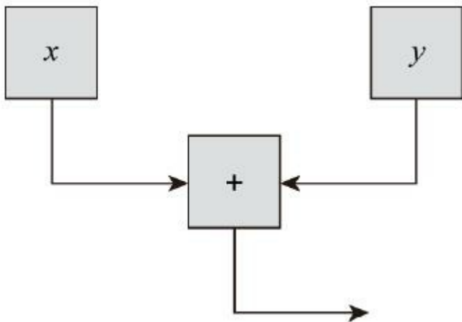
图11-13 构造理想图（1）
