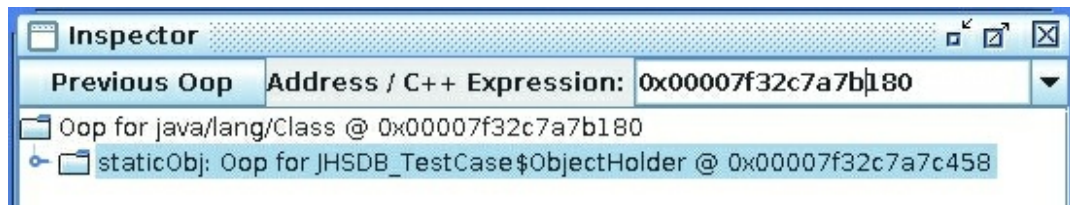
图4-7 Class对象
