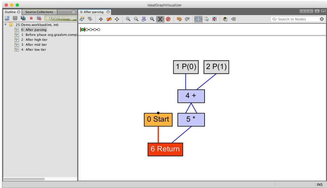
图11-16 构造理想图 (4)
