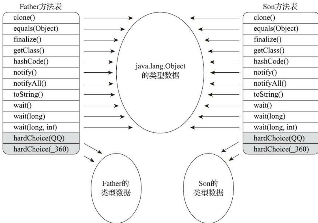
图8-3 方法表结构
